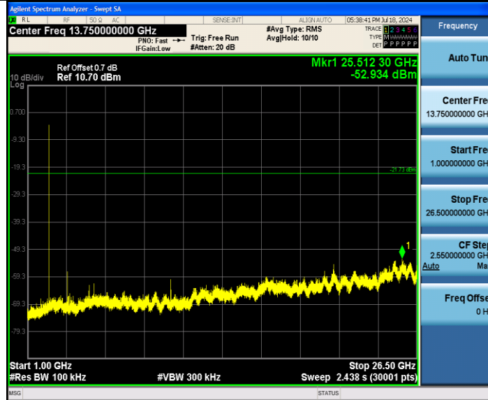
BLE 2M_2440_0~Reference
