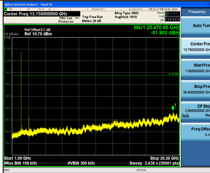
BLE 1M_2480_0~Reference
