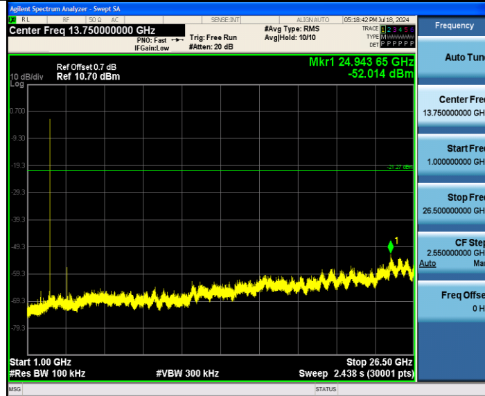
BLE 2M_2402_0~Reference
