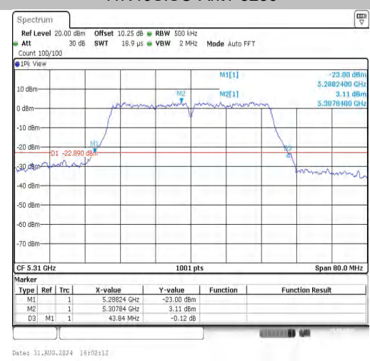
11N40SISO-Ant1-5310
