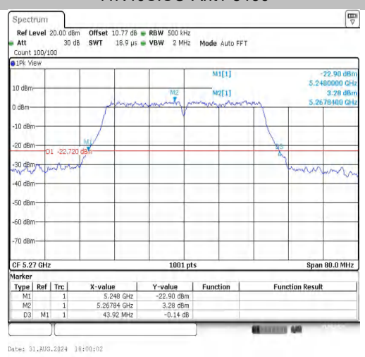
11N40SISO-Ant1-5270
