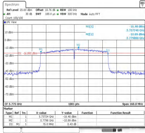
11AC80SISO-Ant1-5775-PASS
