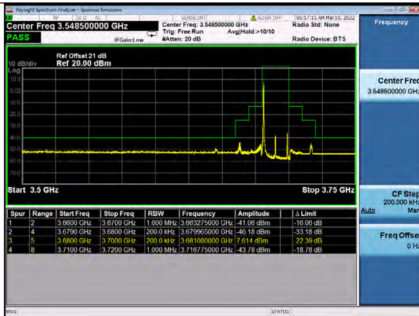
Band48_20MHz_64QAM_HCH_3690MHz_RB_1_99_NTNV
