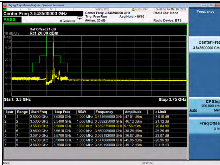
Band48_10MHz_16QAM_LCH_3555MHz_RB_50_0_NTNV
