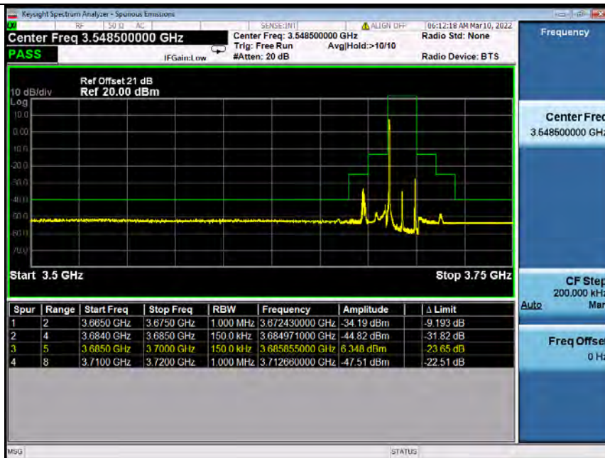
Band48_15MHz_16QAM_HCH_3692.5MHz_RB_1_74_NTNV
