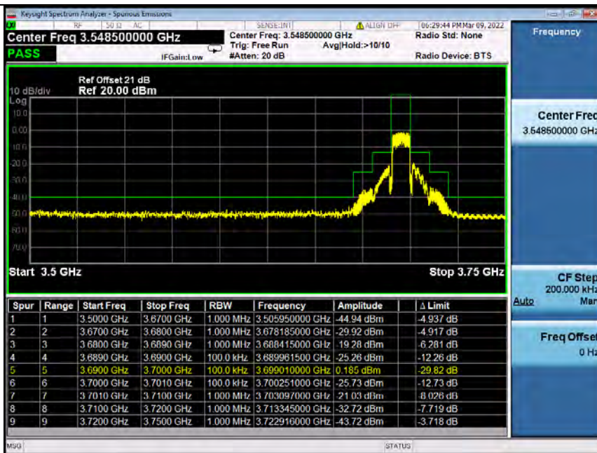
Band48_10MHz_QPSK_HCH_3695MHz_RB_50_0_NTNV
