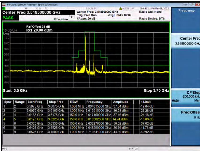
Band48_15MHz_64QAM_MCH_3625MHz_RB_1_74_NTNV
