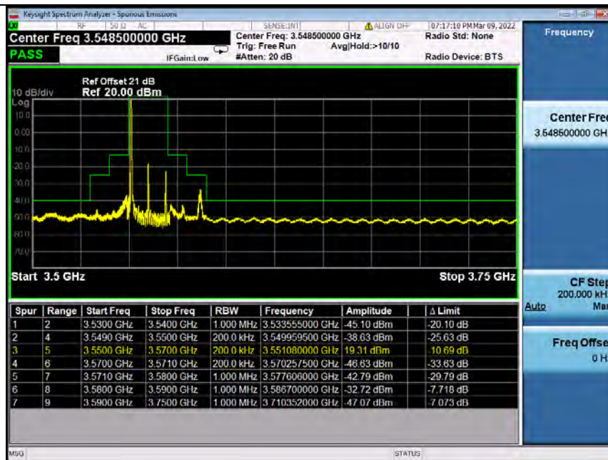
Band48_20MHz_QPSK_LCH_3560MHz_RB_1_99_NTNV
