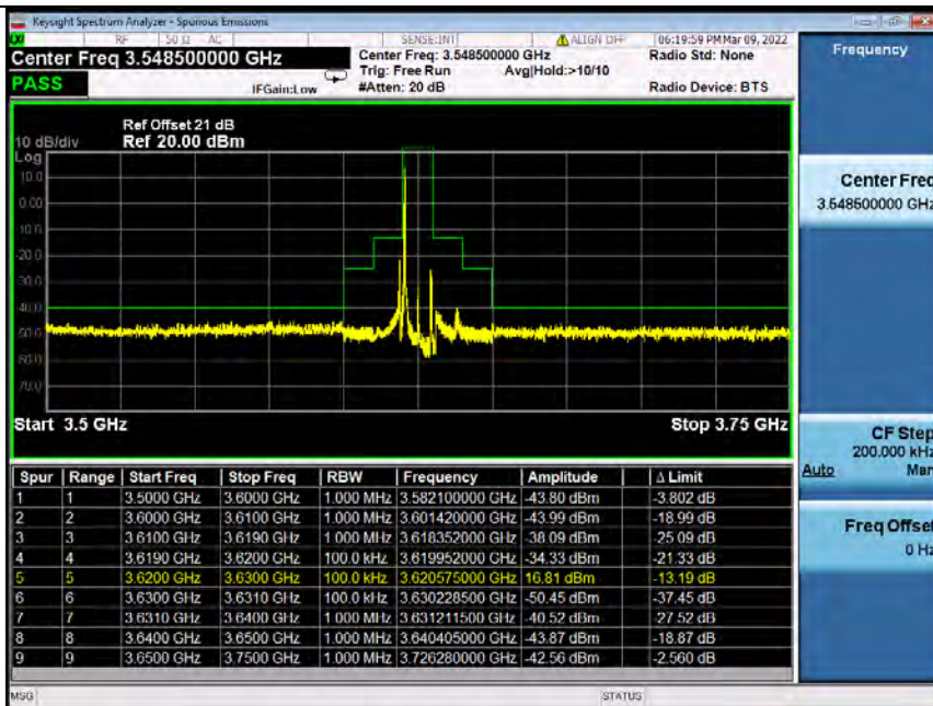
Band48_10MHz_64QAM_MCH_3625MHz_RB_1_49_NTNV
