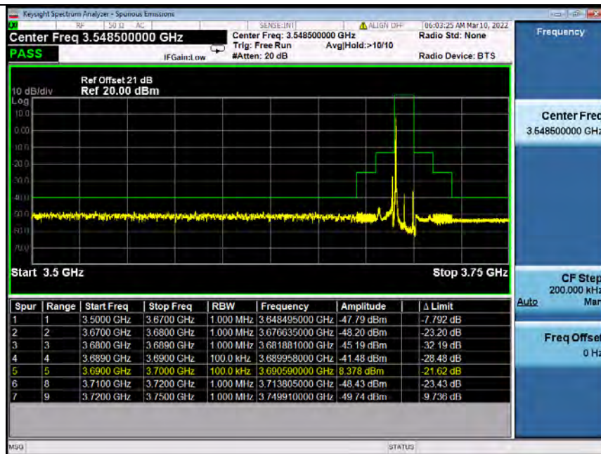
Band48_10MHz_64QAM_HCH_3695MHz_RB_1_49_NTNV
