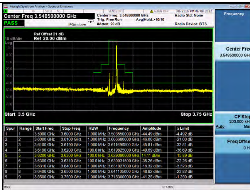
Band48_10MHz_QPSK_MCH_3625MHz_RB_50_0_NTNV
