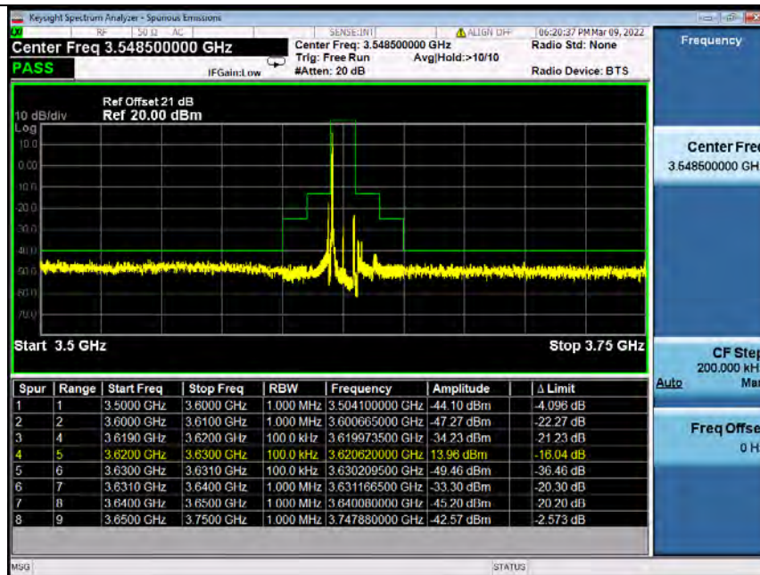
Band48_10MHz_QPSK_MCH_3625MHz_RB_1_49_NTNV
