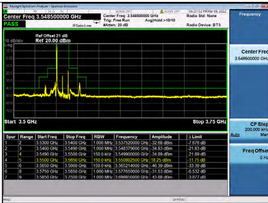
Band48_15MHz_QPSK_LCH_3557.5MHz_RB_1_74_NTNV
