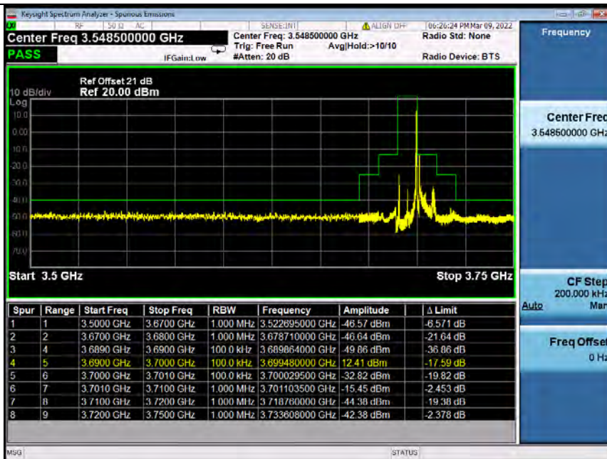
Band48_10MHz_QPSK_HCH_3695MHz_RB_50_0_NTNV
