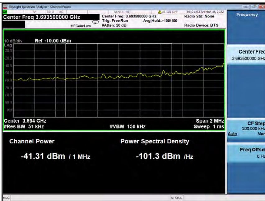
Band48_5MHz_QPSK_HCH_3697.5MHz_RB_1_24_NTNV
