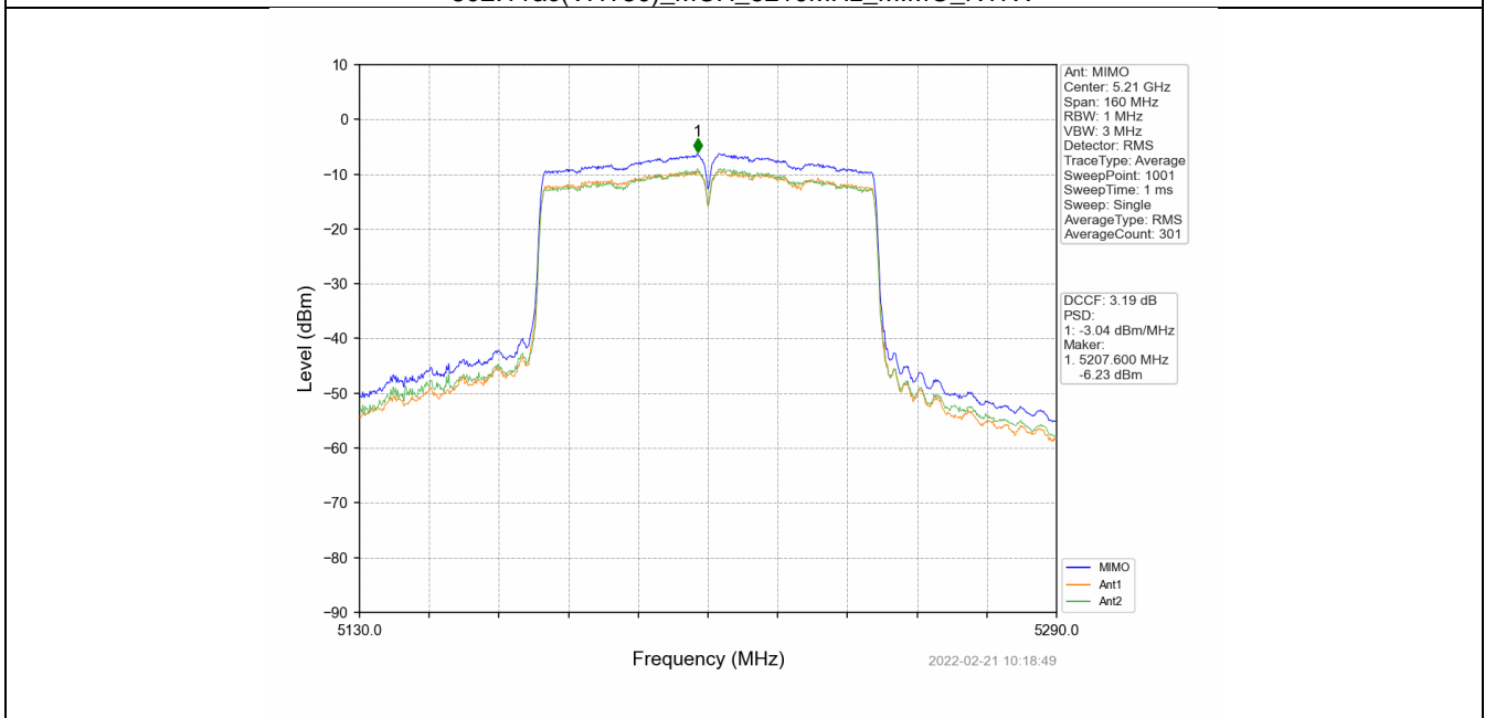
802.11ac(VHT80)_MCH_5210MHz_MIMO_NTNV
