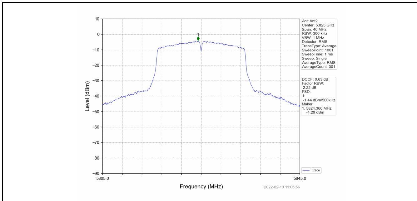
802.11n(HT20)_HCH_5825MHz_MIMO_NTNV
