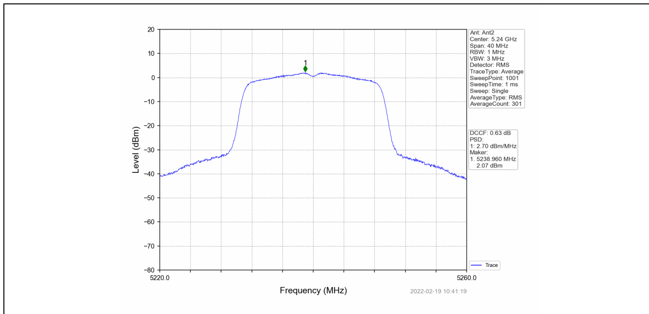
802.11n(HT20)_HCH_5240MHz_MIMO_NTNV
