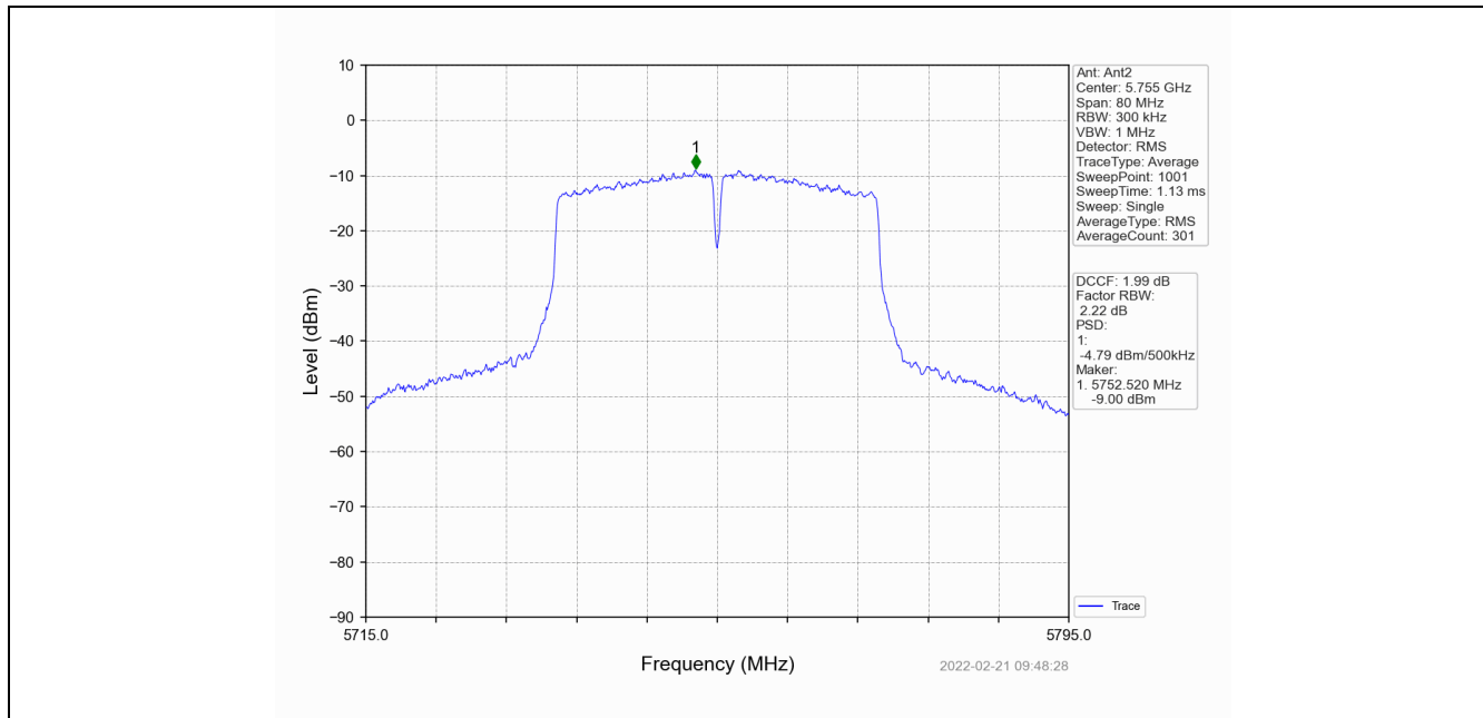
802.11ac(VHT40)_LCH_5755MHz_MIMO_NTNV
