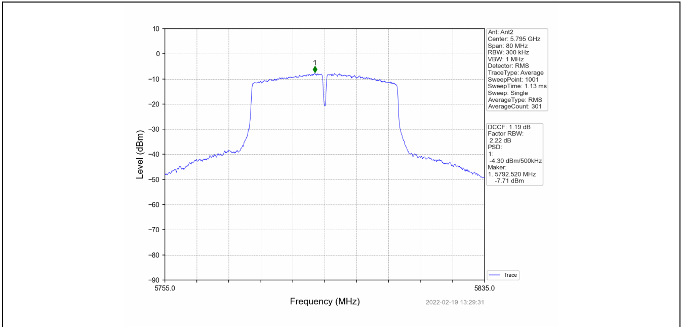
802.11n(HT40)_HCH_5795MHz_MIMO_NTNV
