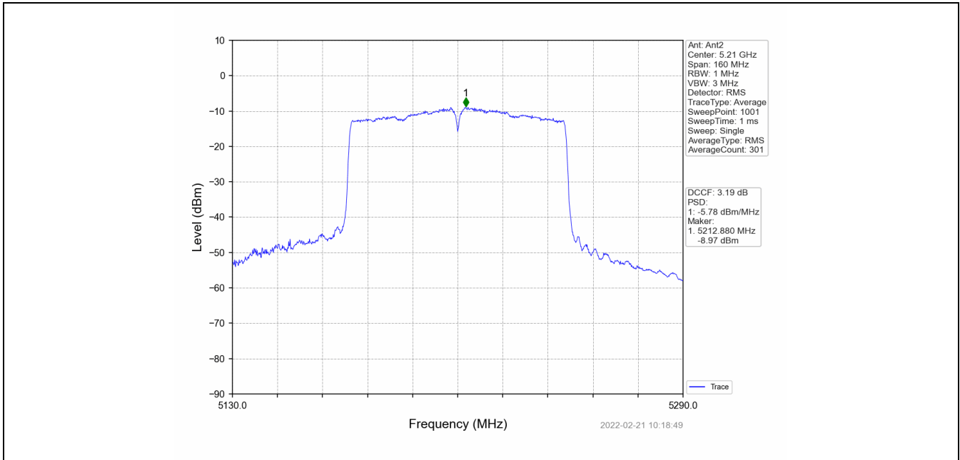
802.11ac(VHT80)_MCH_5210MHz_MIMO_NTNV
