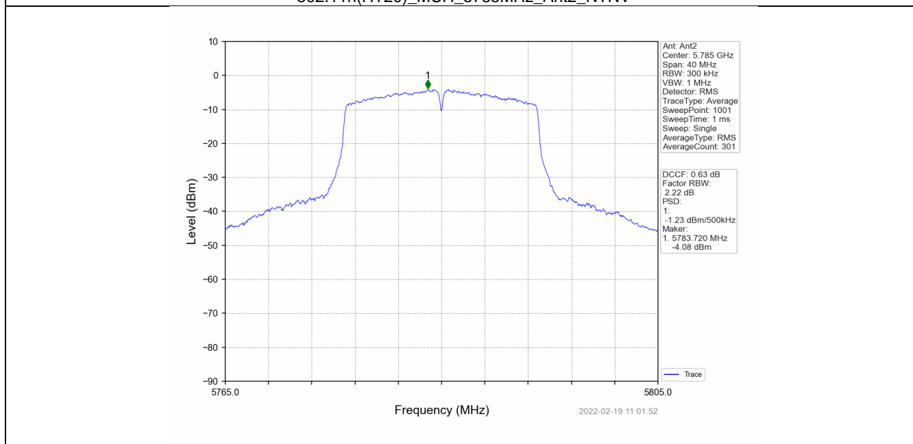
802.11n(HT20)_MCH_5785MHz_MIMO_NTNV
