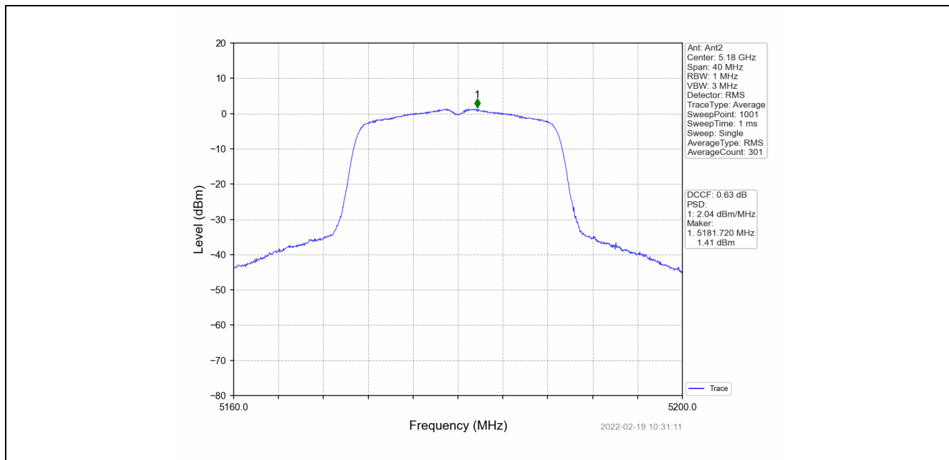
802.11n(HT20)_LCH_5180MHz_MIMO_NTNV
