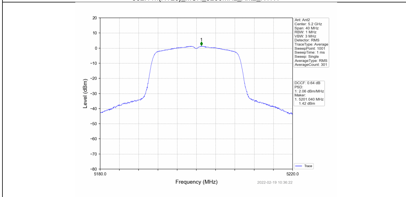
802.11n(HT20)_MCH_5200MHz_MIMO_NTNV
