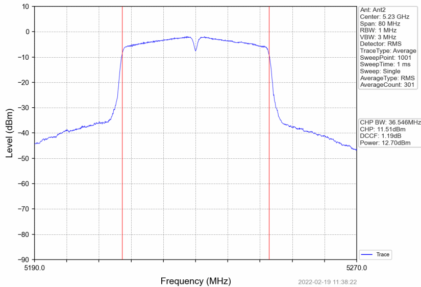
802.11n(HT40)_HCH_5230MHz_Ant2_NTNV
