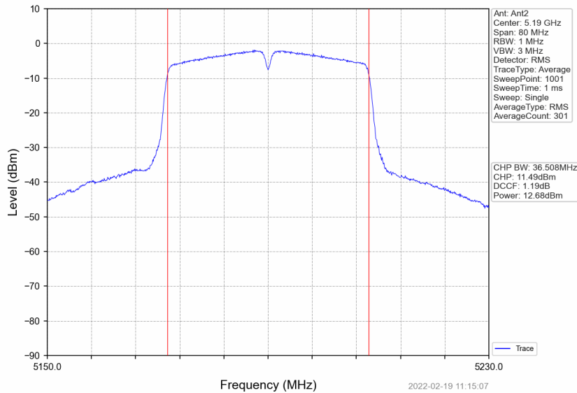
802.11n(HT40)_LCH_5190MHz_Ant2_NTNV
