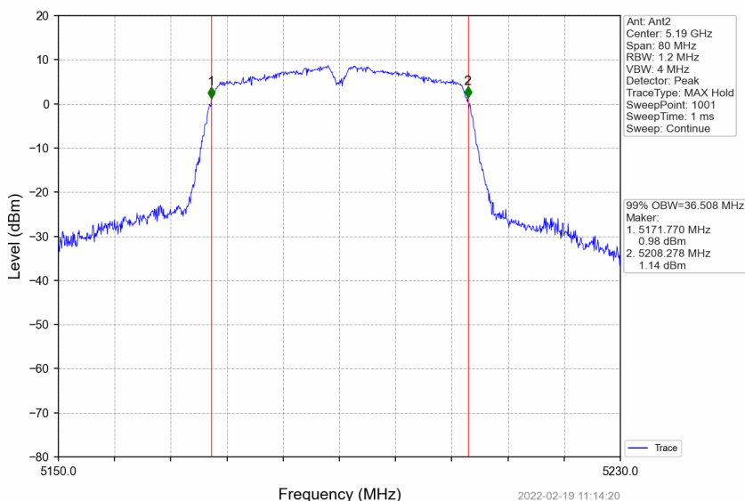
802.11n(HT40)_LCH_5190MHz_Ant2_NTNV
