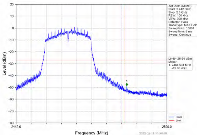
802.11n(HT20)_HCH_2462MHz_Ant1 (MIMO)_NTNV
