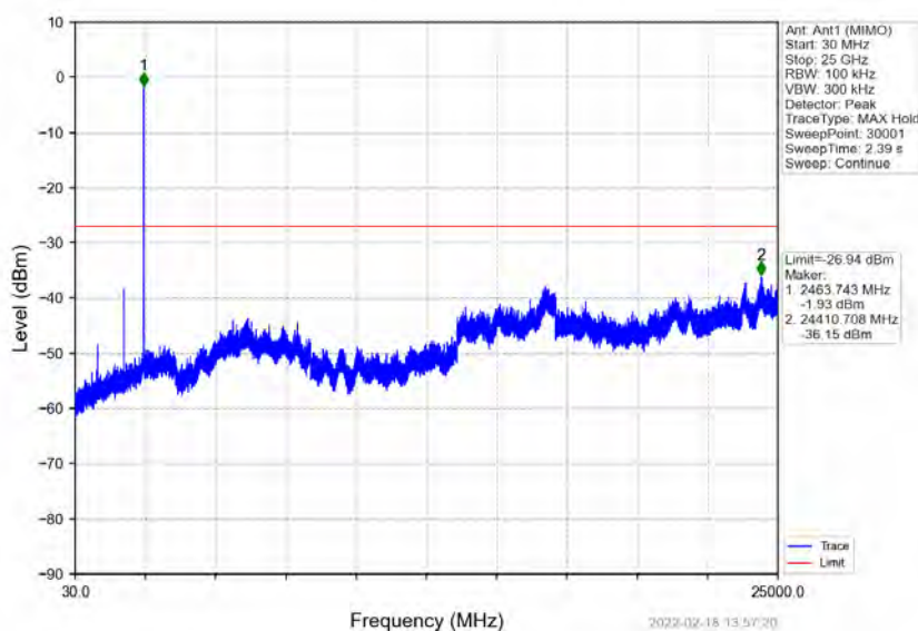
802.11n(HT20)_HCH_2462MHz_Ant1 (MIMO)_NTNV
