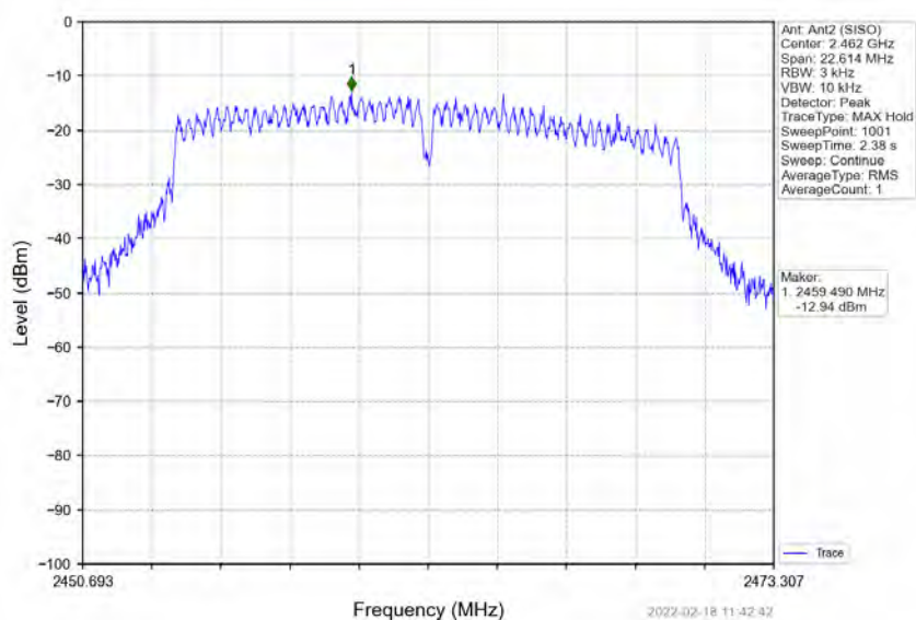
802.11g_HCH_2462MHz_Ant2 (SISO)_NTNV
