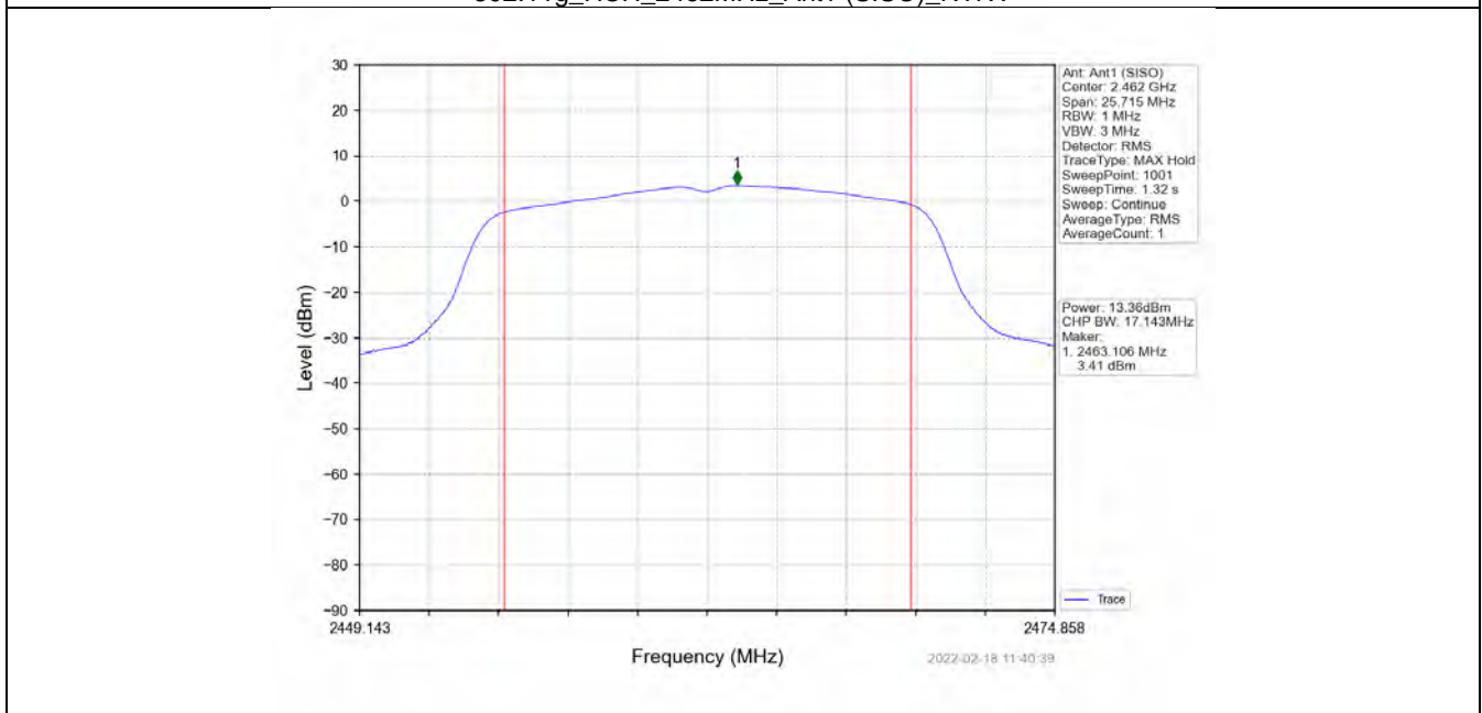
802.11g_HCH_2462MHz_Ant2 (SISO)_NTNV
