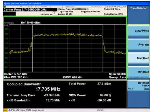
16QAM, CH53140
