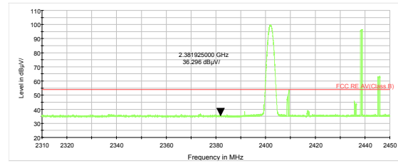
BLE Channel 0 Average
