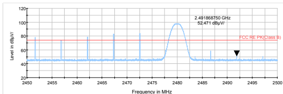
BLE Channel 39 Peak
