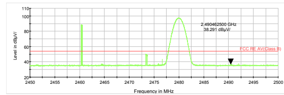
BLE Channel 39 Average
