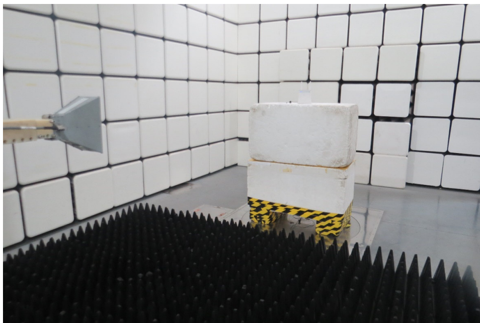
1GHz-18GHz
