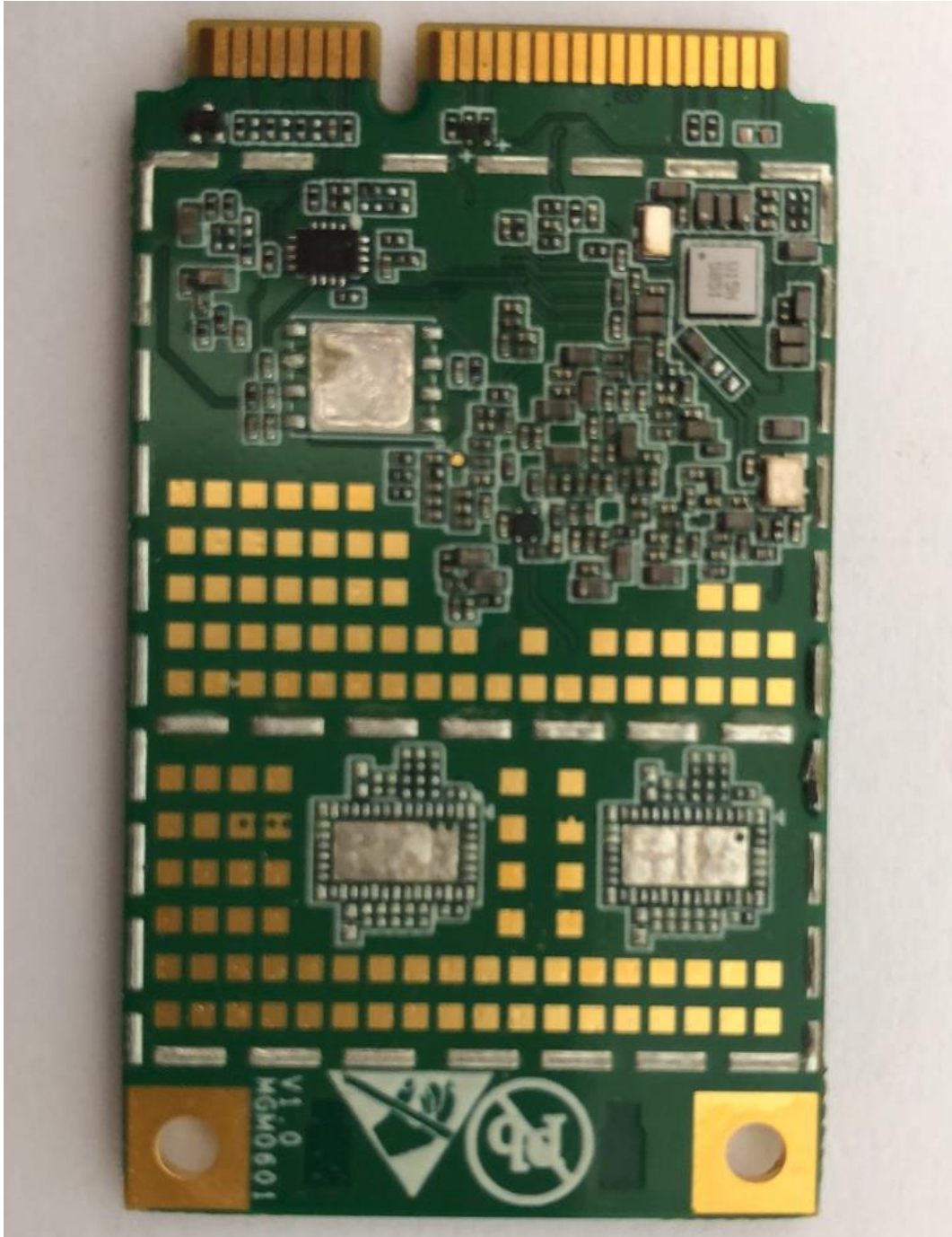
a: EUT
