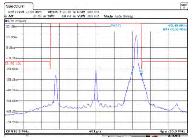
LTE Band 26 QPSK 10MHz CH-High 1RB
