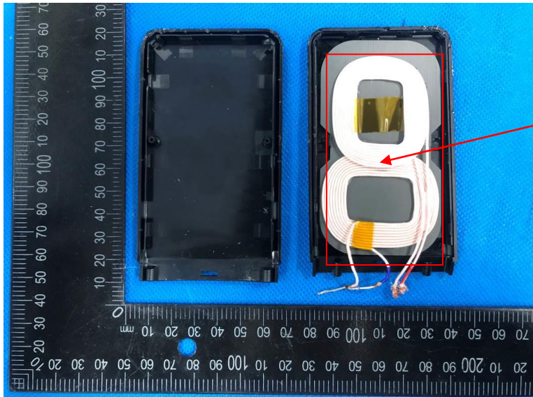
ANTENNA
