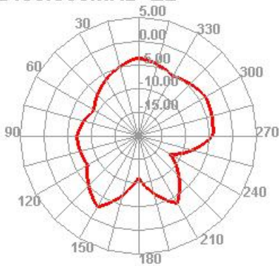
2480.000MHz E2
