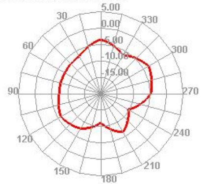
2480.000MHz E1
