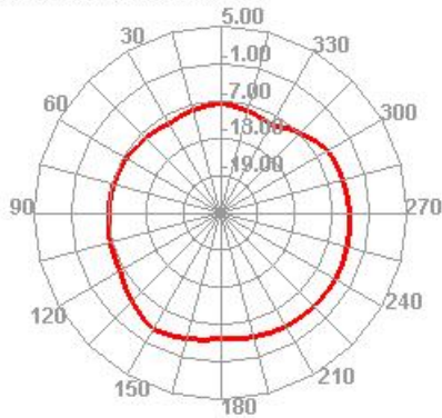
2480.000MHz H
