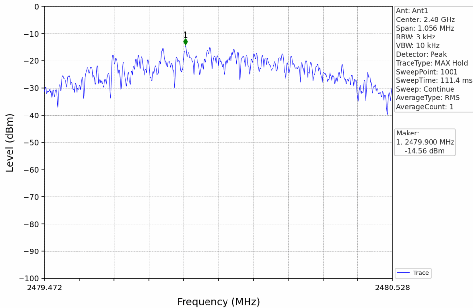
1M_HCH_2480MHz_DataRate=_Ant1_NTNV
