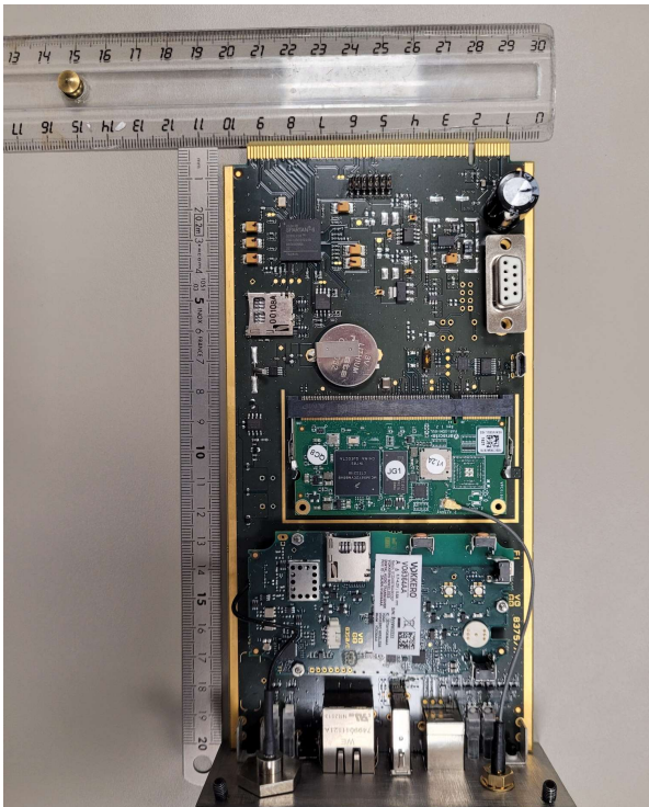
Module VO8364A Up
