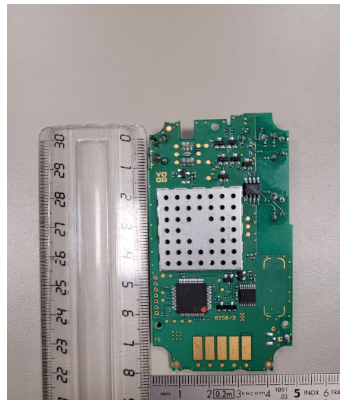
Module VO8364A Bottom
