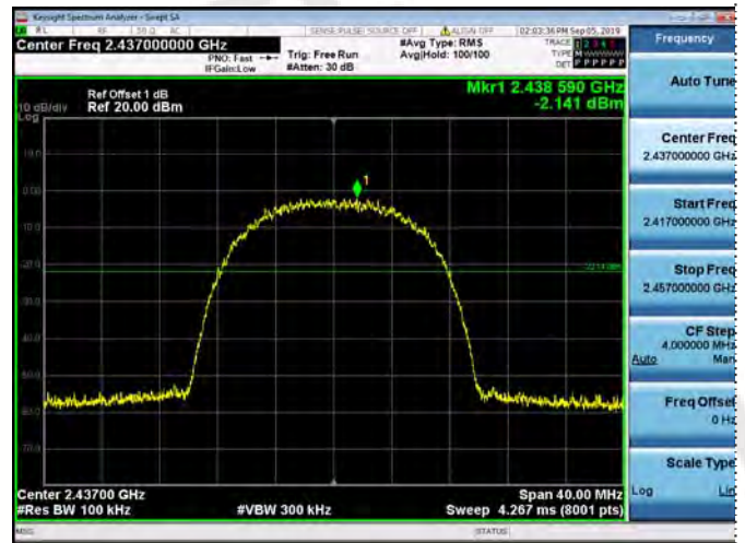
802.11b CH06
