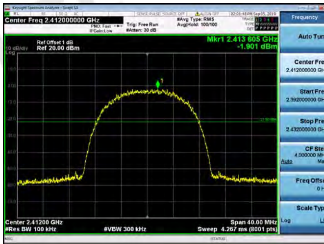
802.11b CH01
