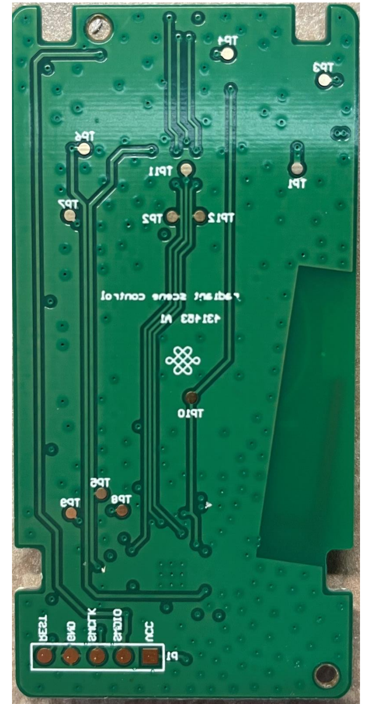
PCBA - BOT
