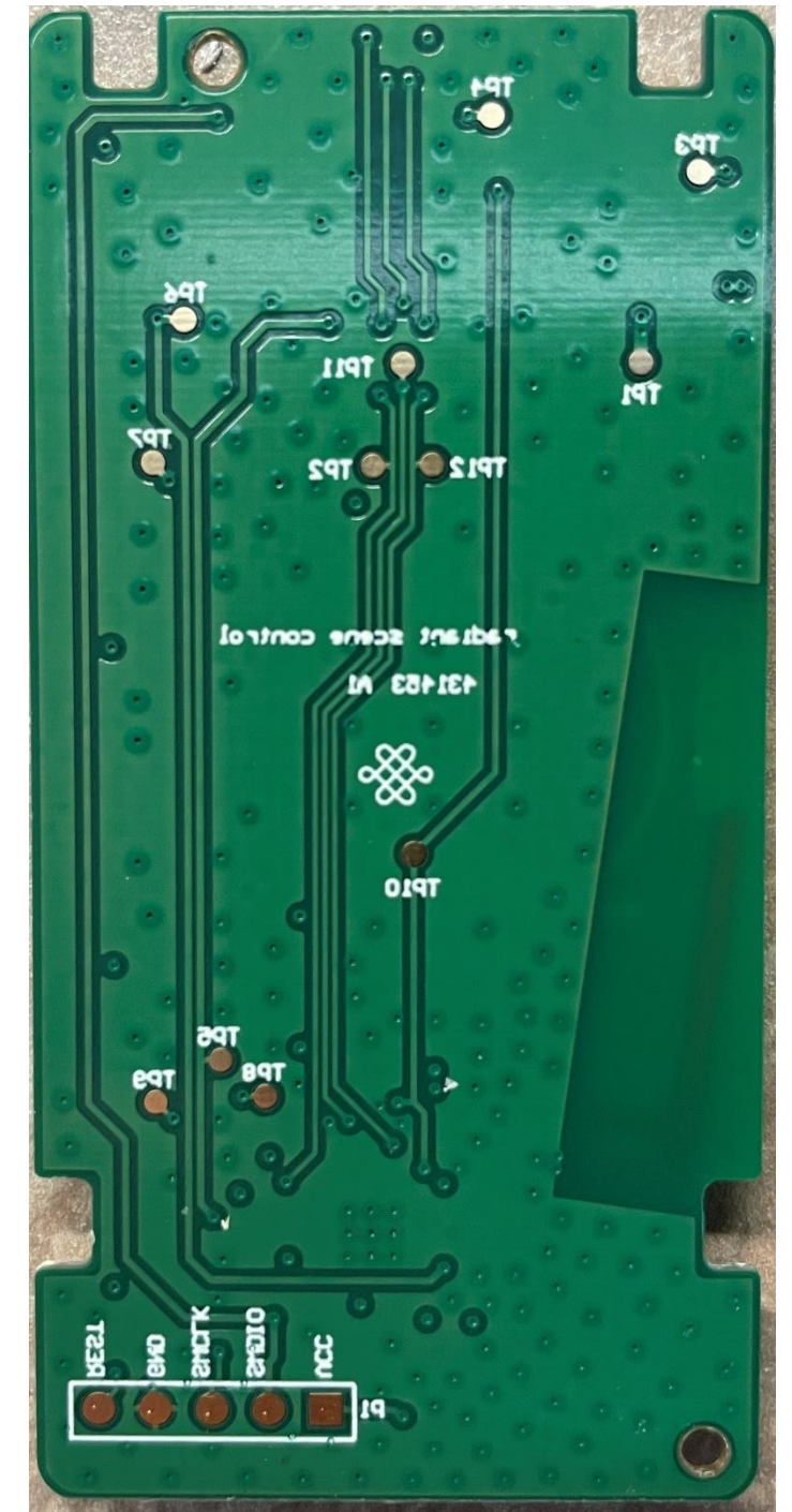
PCBA - BOT
