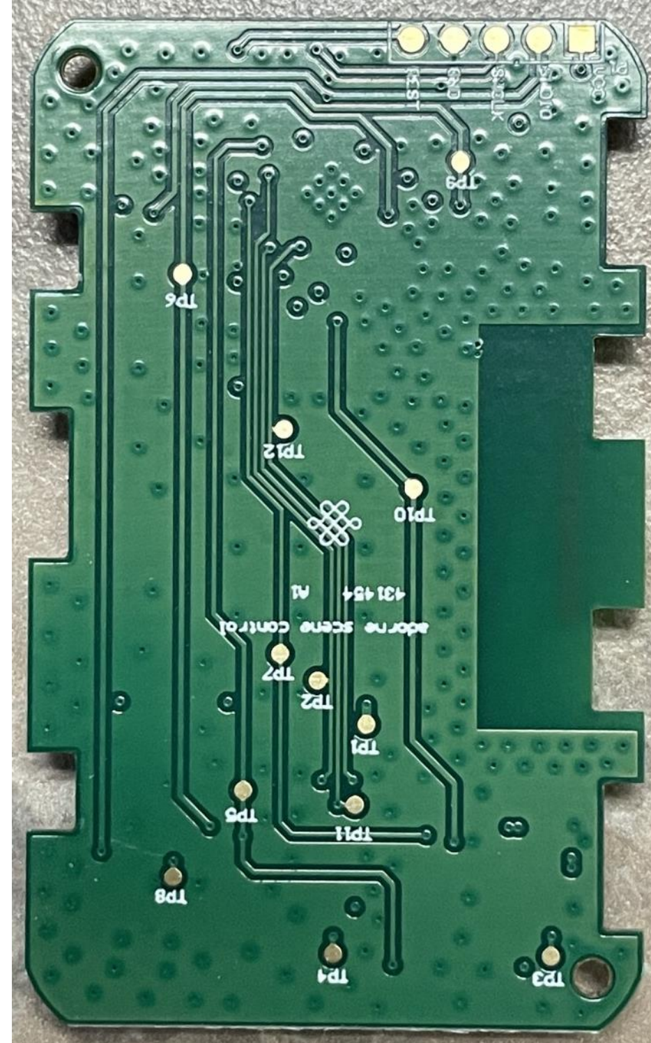
PCBA - BOT
