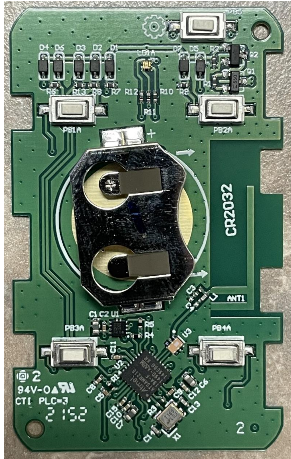
PCBA - TOP
