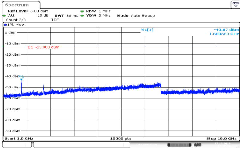
Band5-10MHz-QPSK-20600-50RB#0-Range4:1000~10000MHz
