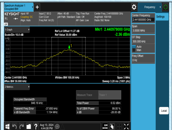
DH5-Ant1-2441
