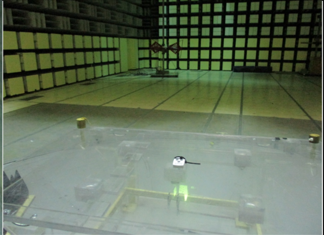
EUT RE 30MHz - 1GHz
