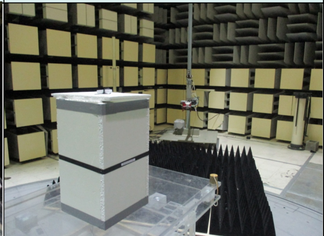
EUT RE 1GHz - 5GHz
