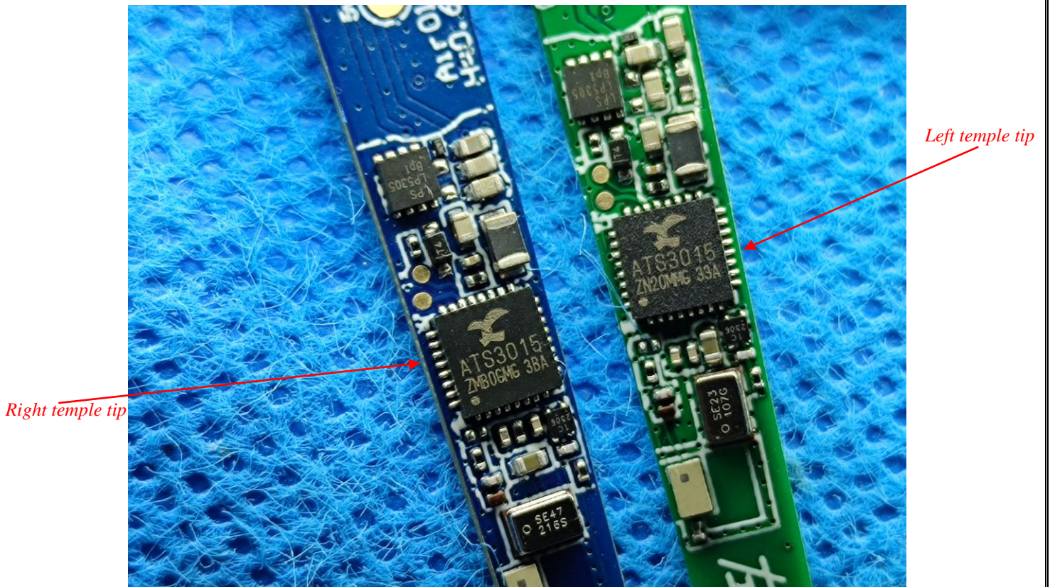
Antenna
