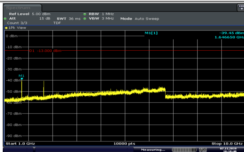
Band26-3MHz-QPSK-26775-15RB#0-Range4:1000~10000MHz
