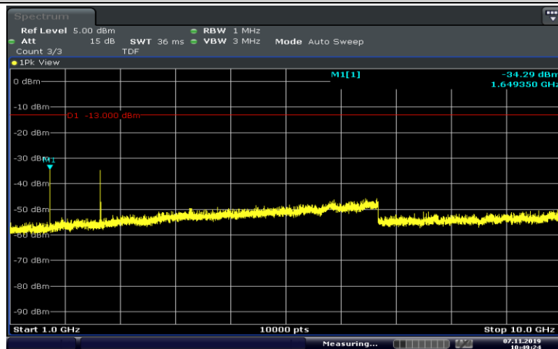
Band26-1.4MHz-QPSK-26797-6RB#0-Range4:1000~10000MHz
