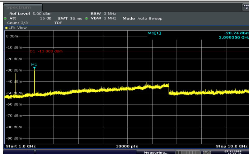
Band12-1.4MHz-QPSK-23017-6RB#0-Range2:1000~10000MHz
