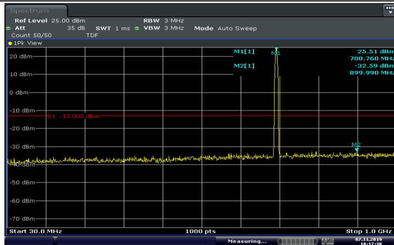
Band12-1.4MHz-QPSK-23017-6RB#0-Range1:30~1000MHz
