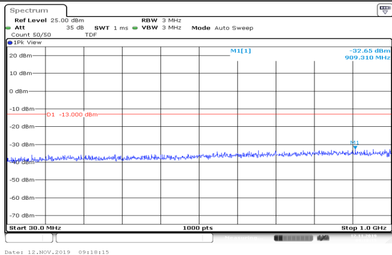
Band4-10MHz-QPSK-20000-50RB#0-Range3:30~1000MHz
