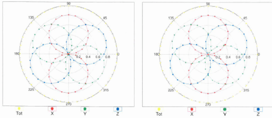
f=1800 MHz,R22
