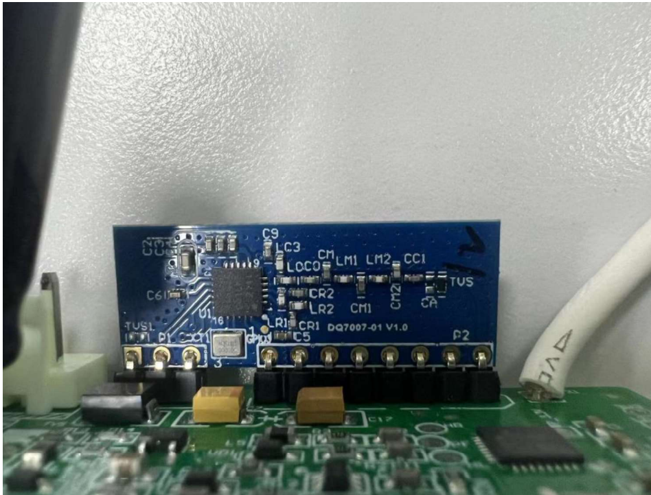
RF Module
