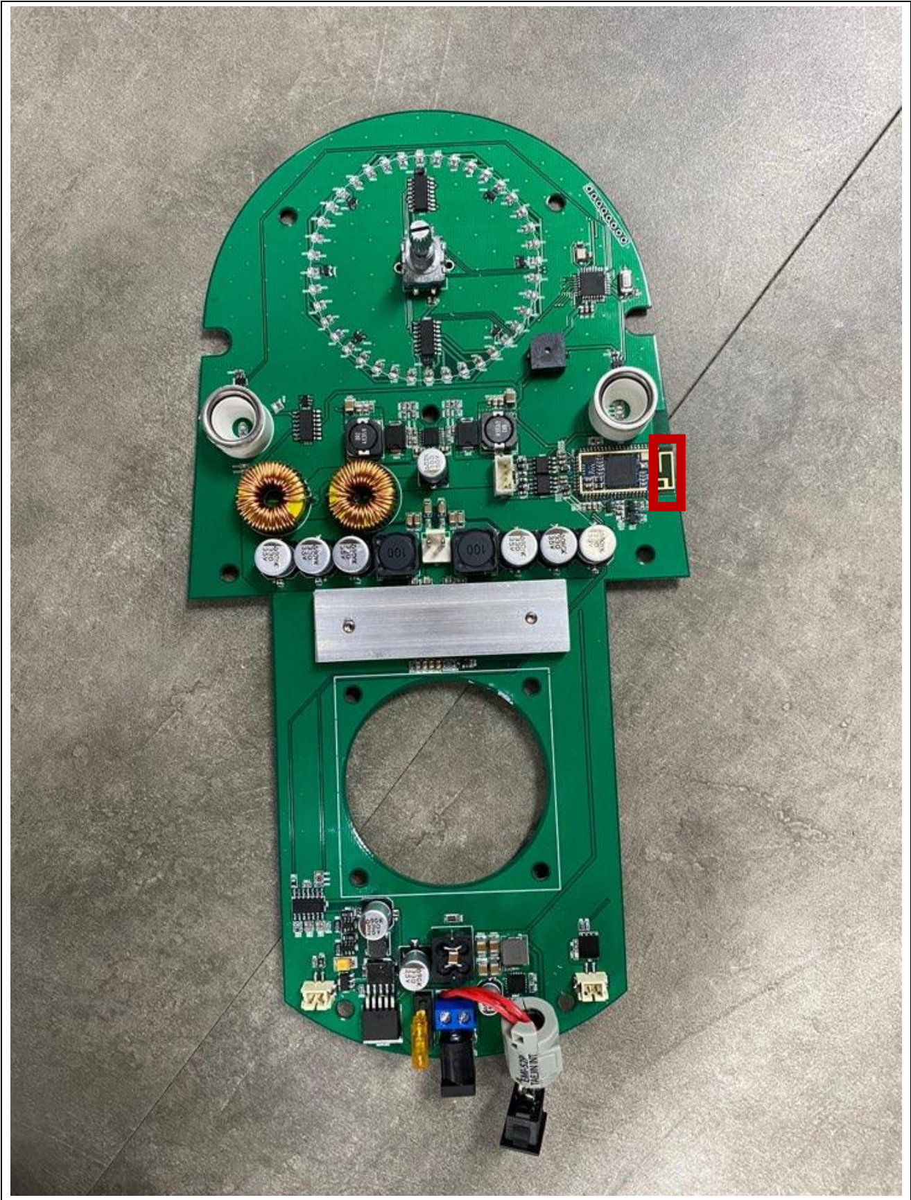
Antenna
