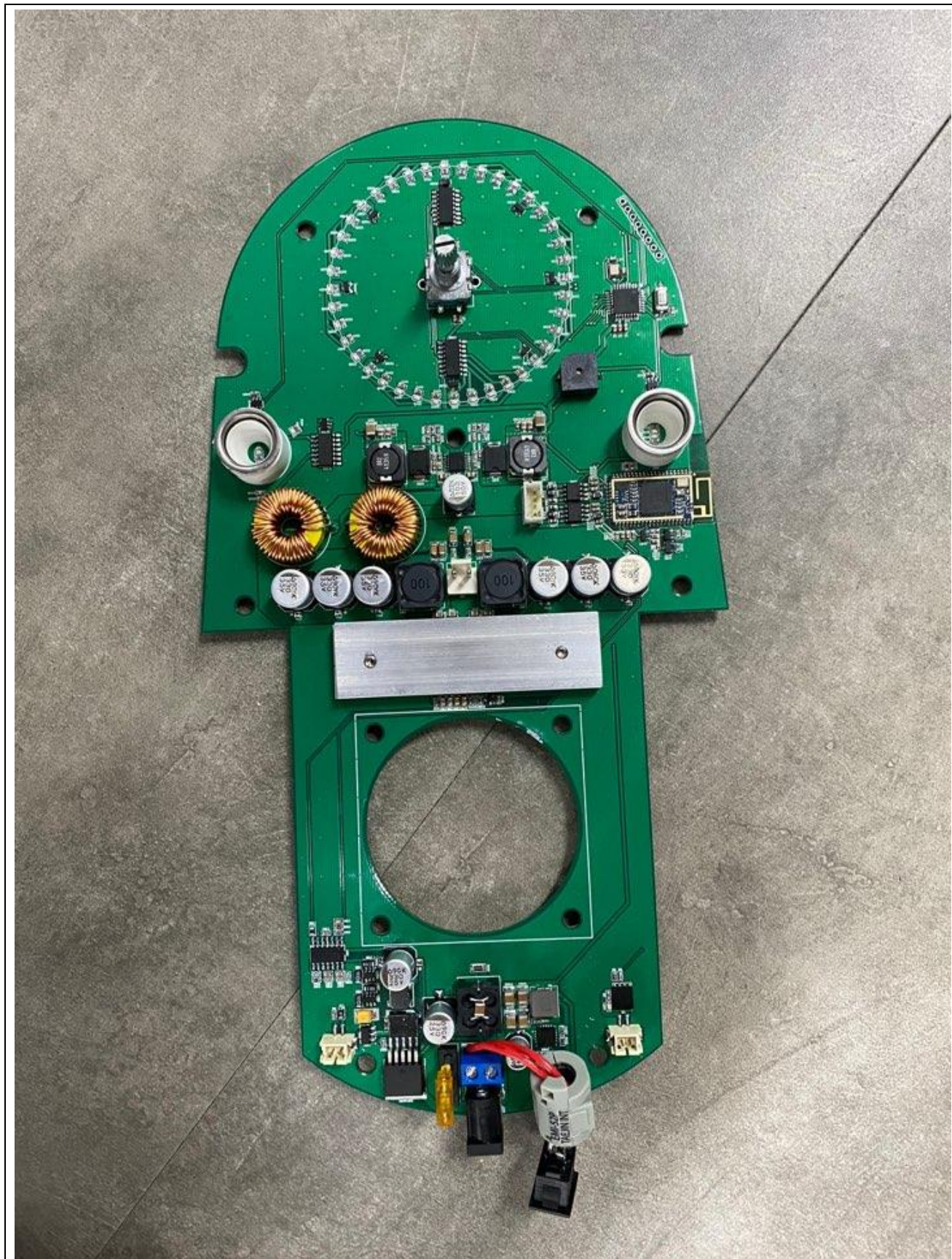
MainBoard-Front
