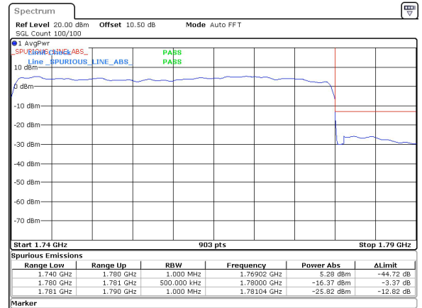
40MHz_15kHz_1760MHz_DFT-s-OFDM QPSK_RB216@0&-16.37 dBm
