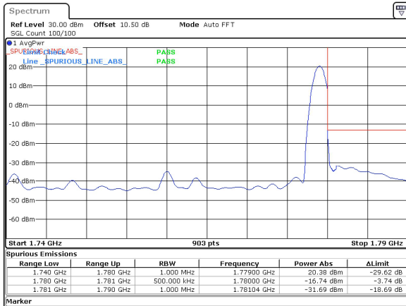
40MHz_15kHz_1760MHz_DFT-s-OFDM QPSK_RB1@215&-16.74 dBm
