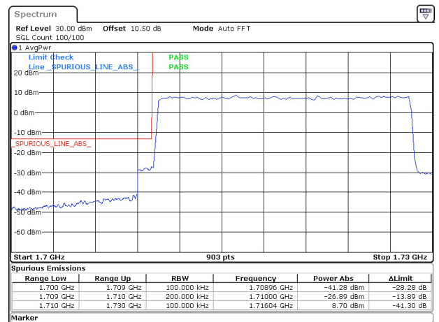
20MHz_15kHz_1720MHz_DFT-s-OFDM QPSK_RB100@0&-26.89 dBm
