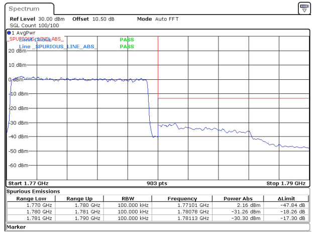
10MHz_15kHz_1775MHz_DFT-s-OFDM QPSK_RB50@0&-30.30 dBm
