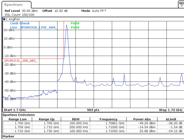
20MHz_15kHz_1720MHz_DFT-s-OFDM QPSK_RB1@0&-14.54 dBm
