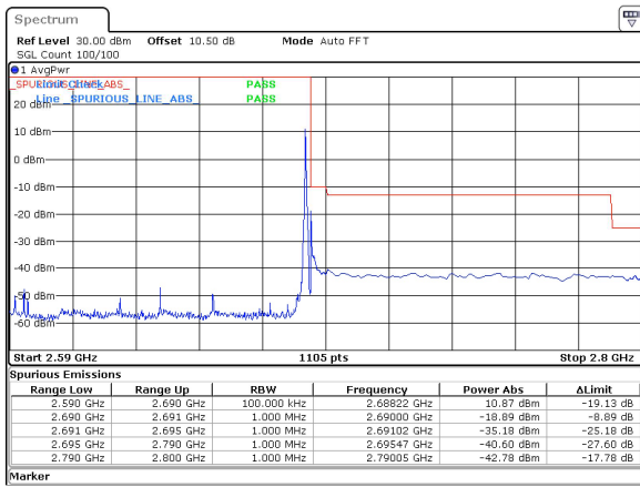
100MHz_30kHz_2640MHz_DFT-s-OFDM QPSK_RB1@272&-18.89 dBm
