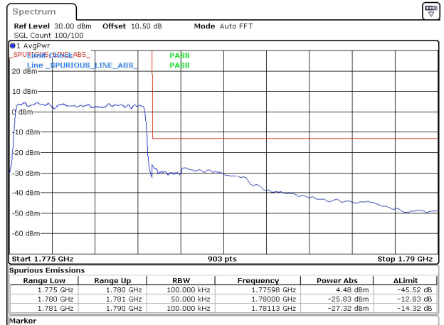
5MHz_15kHz_1777.5MHz_DFT-s-OFDM QPSK_RB25@0&-25.83 dBm
