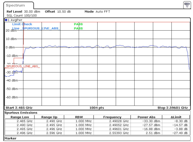
100MHz_30kHz_2546.01MHz_DFT-s-OFDM QPSK_RB270@0&-16.88 dBm
