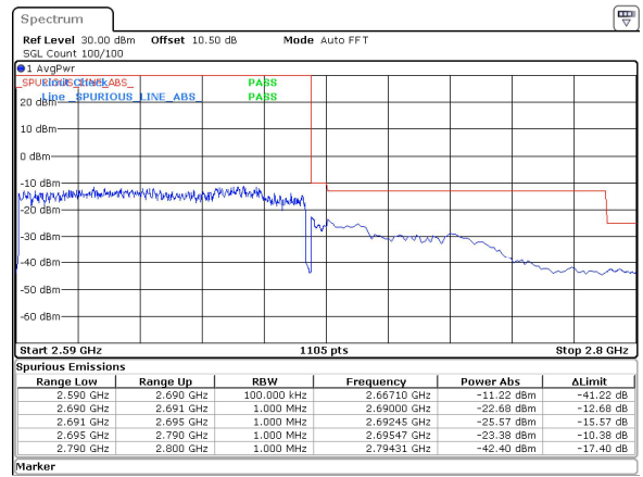
100MHz_30kHz_2640MHz_DFT-s-OFDM QPSK_RB270@0&-23.38 dBm
