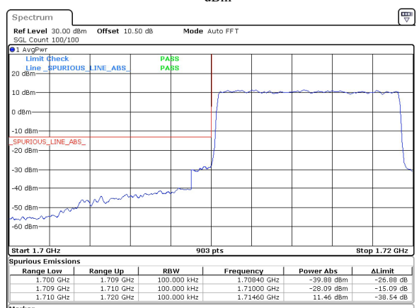
10MHz_15kHz_1715MHz_DFT-s-OFDM QPSK_RB50@0&-28.09 dBm
