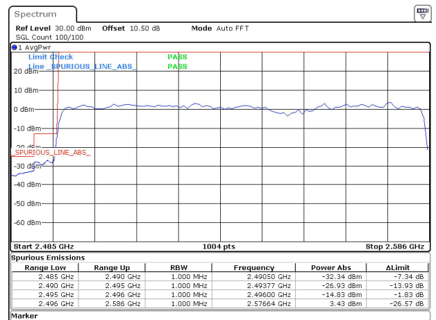
90MHz_30kHz_2541MHz_DFT-s-OFDM QPSK_RB243@0~-14.83 dBm
