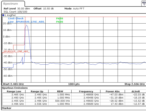
60MHz_30kHz_2526MHz_DFT-s-OFDM QPSK_RB1@0&17.43 dBm
