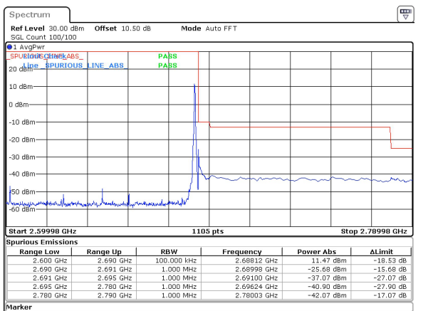
90MHz_30kHz_2644.98MHz_DFT-s-OFDM QPSK_RB1@244~-25.68 dBm
