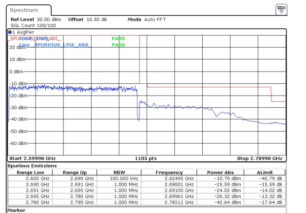
90MHz_30kHz_2644.98MHz_DFT-s-OFDM QPSK_RB243@0~-26.32 dBm
