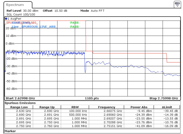
60MHz_30kHz_2659.98MHz_DFT-s-OFDM QPSK_RB162@0&-23.76 dBm
