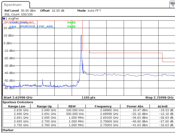
60MHz_30kHz_2659.98MHz_DFT-s-OFDM QPSK_RB1@161&-22.10 dBm
