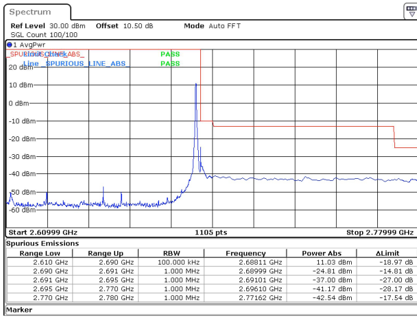
80MHz_30kHz_2649.99MHz_DFT-s-OFDM QPSK_RB1@216~-24.81 dBm
