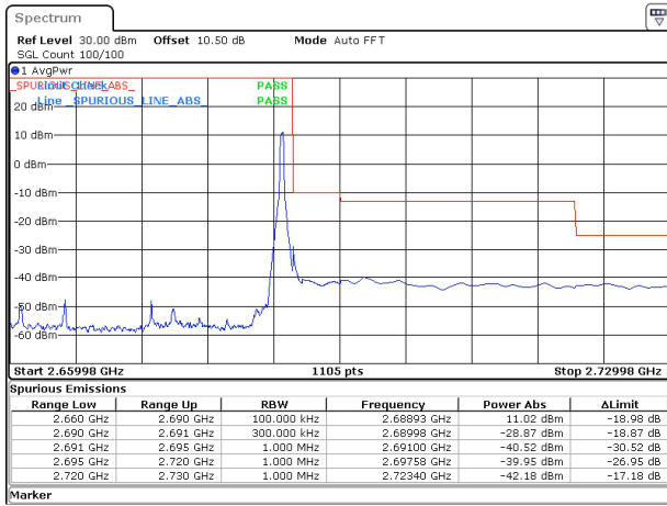
30MHz_30kHz_2674.98MHz_DFT-s-OFDM QPSK_RB1@77&-42.18 dBm
