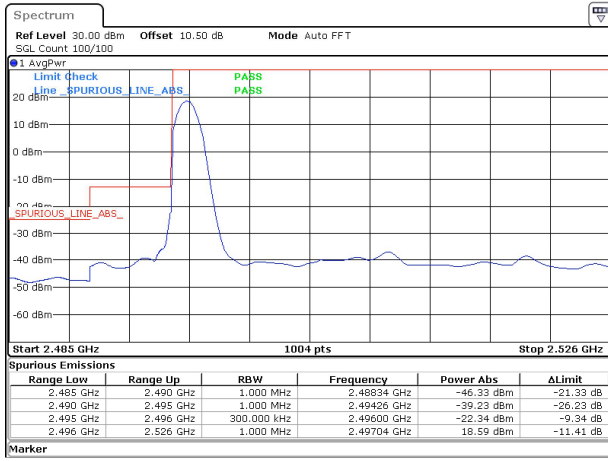
30MHz_30kHz_2511MHz_DFT-s-OFDM QPSK_RB1@0&-22.34 dBm
