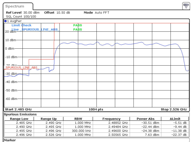
30MHz_30kHz_2511MHz_DFT-s-OFDM QPSK_RB75@0&-30.51 dBm
