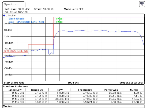
20MHz_30kHz_2506.02MHz_DFT-s-OFDM QPSK_RB50@0&-29.03 dBm
