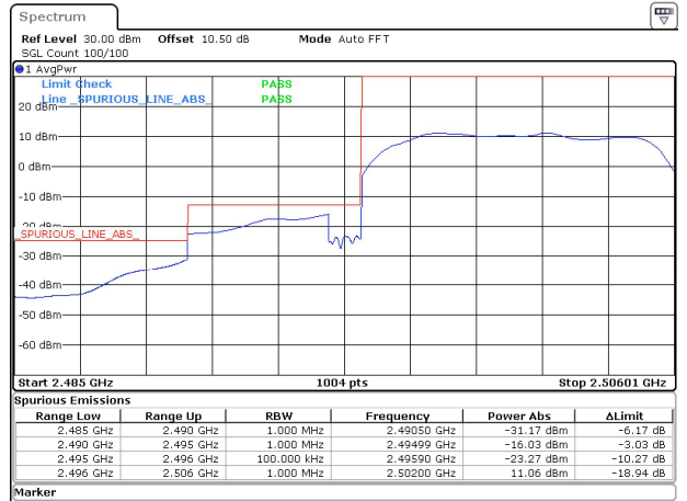
10MHz_30kHz_2501.01MHz_DFT-s-OFDM QPSK_RB24@0&-16.03 dBm
