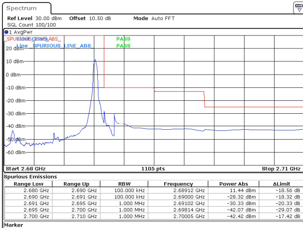
10MHz_30kHz_2685MHz_DFT-s-OFDM QPSK_RB1@23&-42.42 dBm
