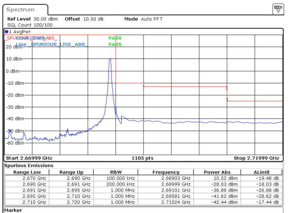
20MHz_30kHz_2679.99MHz_DFT-s-OFDM QPSK_RB1@50&-42.44 dBm
