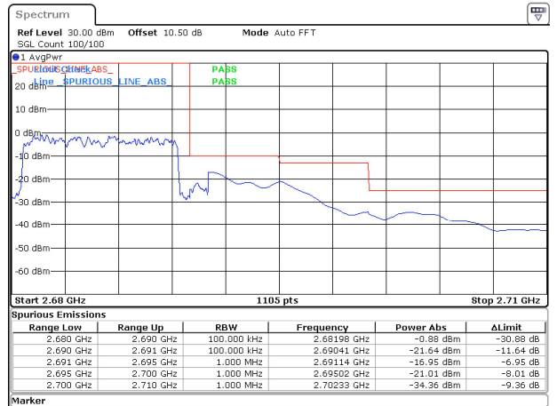
10MHz_30kHz_2685MHz_DFT-s-OFDM QPSK_RB24@0&-16.95 dBm
