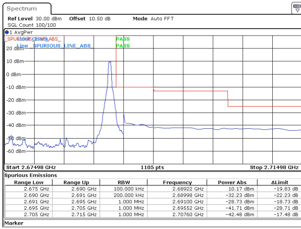
15MHz_30kHz_2682.48MHz_DFT-s-OFDM QPSK_RB1@37&-42.48 dBm
