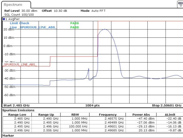
10MHz_30kHz_2501.01MHz_DFT-s-OFDM QPSK_RB1@0&20.13 dBm
