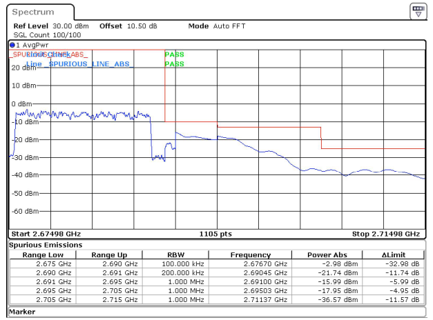
15MHz_30kHz_2682.48MHz_DFT-s-OFDM QPSK_RB36@0&-17.95 dBm
