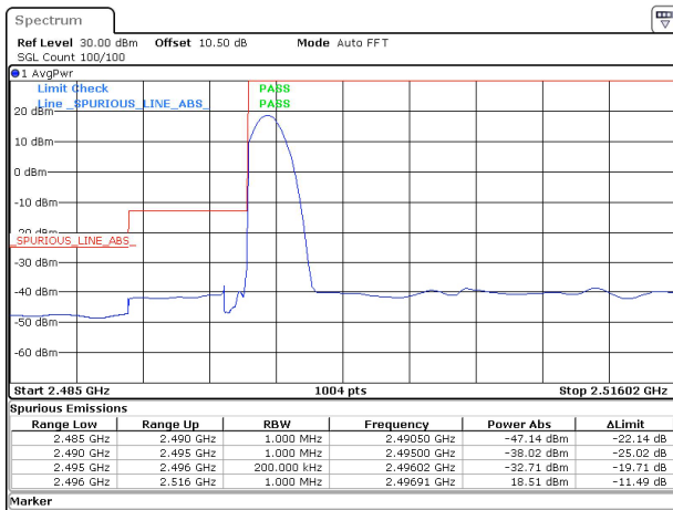
20MHz_30kHz_2506.02MHz_DFT-s-OFDM QPSK_RB1@0&18.51 dBm
