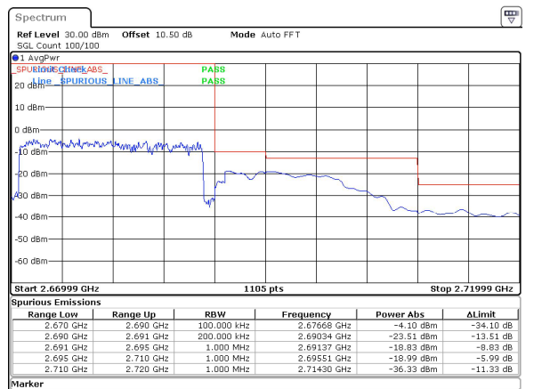
20MHz_30kHz_2679.99MHz_DFT-s-OFDM QPSK_RB50@0&-18.99 dBm
