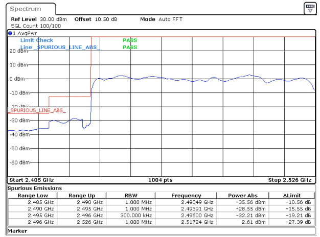
10MHz|30MHz 15kHz 1880MHz|2511MHz DFT-s-OFDM QPSK_RB0|RB160@0&-35.56 dBm
