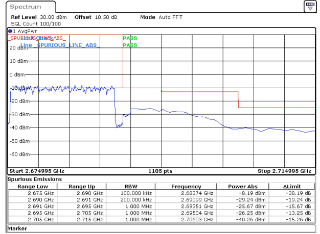
10MHz|15MHz_15kHz_1880MHz|2682.495MHz_DFT-s-OFDM QPSK_RB0|RB75@0&-26.25 dBm
