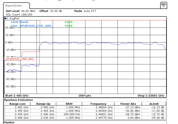
10MHz|40MHz 15kHz 1880MHz|2516.01MHz DFT-s-OFDM QPSK_RB0|RB216@0&-37.13 dBm
