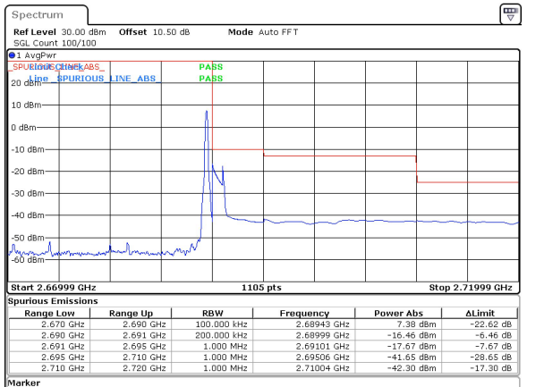
10MHz|20MHz_15kHz_1880MHz|2679.99MHz_DFT-s-OFDM QPSK_RB0|RB1@105&-16.46 dBm
