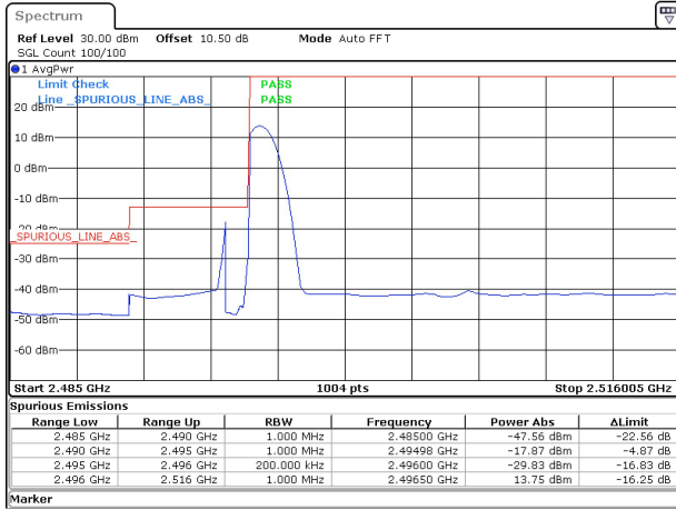
10MHz|20MHz_15kHz_1880MHz|2506.005MHz_DFT-s-OFDM QPSK_RB0|RB1@0&-17.87 dBm
