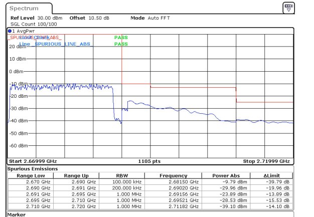
10MHz|20MHz_15kHz_1880MHz|2679.99MHz_DFT-s-OFDM QPSK_RB0|RB100@0&-23.89 dBm
