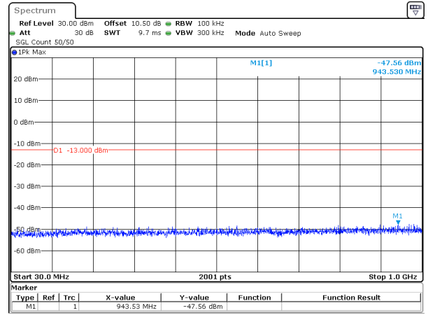
20MHz_15kHz_1770MHz_DFT-s-OFDM QPSK_RB1@0&-47.56 dBm
