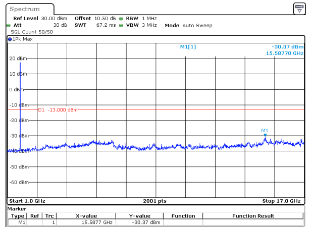
10MHz_15kHz_1715MHz_DFT-s-OFDM QPSK_RB50@0&-30.37 dBm
