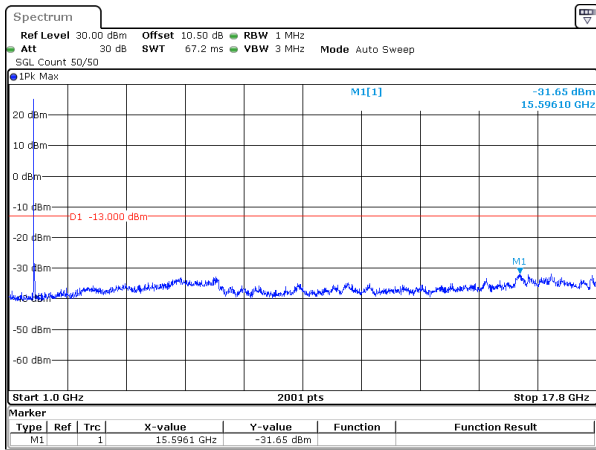
20MHz_15kHz_1720MHz_DFT-s-OFDM QPSK_RB1@0&-31.65 dBm
