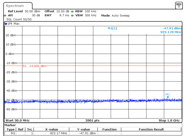
5MHz_15kHz_1712.5MHz_DFT-s-OFDM QPSK_RB25@0&-47.91 dBm
