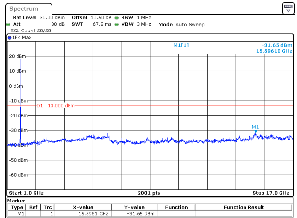
10MHz_15kHz_1775MHz_DFT-s-OFDM QPSK_RB50@0&-31.65 dBm
