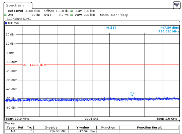
20MHz_15kHz_1770MHz_DFT-s-OFDM QPSK_RB100@0&-47.59 dBm
