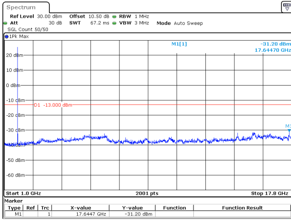
20MHz_15kHz_1770MHz_DFT-s-OFDM QPSK_RB1@0&-31.20 dBm
