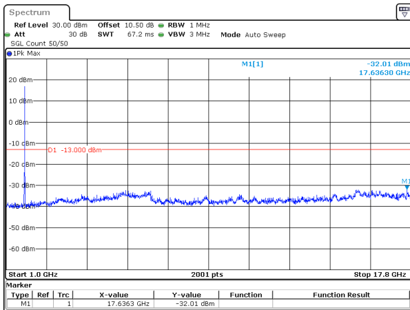
20MHz_15kHz_1770MHz_DFT-s-OFDM QPSK_RB100@0&-32.01 dBm
