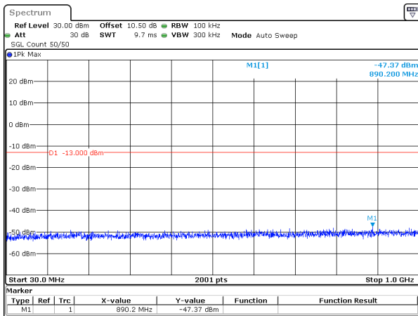
10MHz_15kHz_1715MHz_DFT-s-OFDM QPSK_RB50@0&-47.37 dBm
