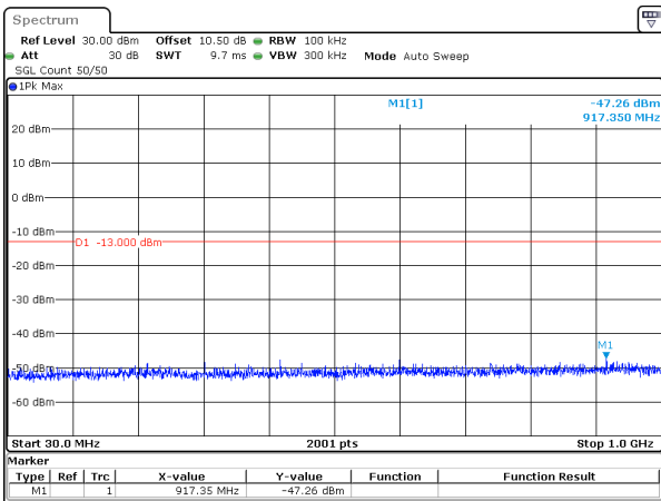
10MHz_15kHz_1745MHz_DFT-s-OFDM QPSK_RB50@0&-47.26 dBm
