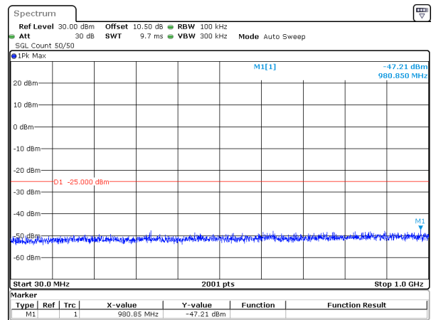
100MHz_30kHz_2640MHz_DFT-s-OFDM QPSK_RB1@272&-47.21 dBm
