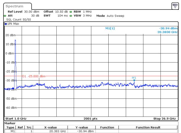
100MHz_30kHz_2640MHz_DFT-s-OFDM QPSK_RB270@0&-30.94 dBm
