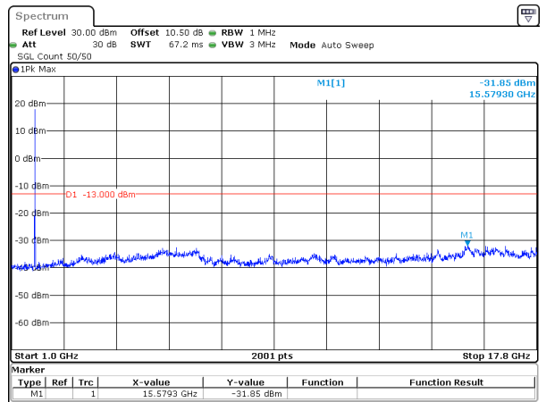
10MHz_15kHz_1745MHz_DFT-s-OFDM QPSK_RB50@0&-31.85 dBm
