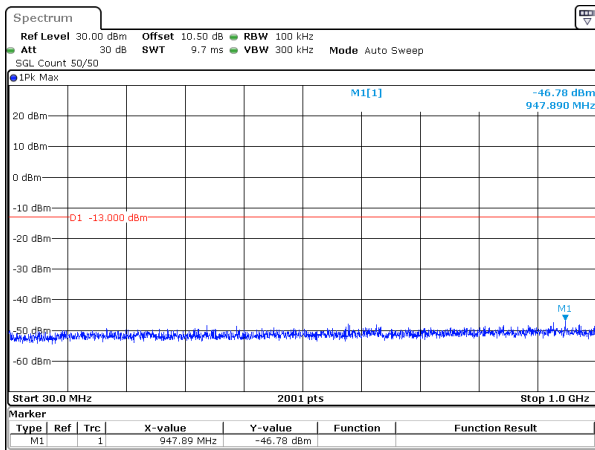
10MHz_15kHz_1775MHz_DFT-s-OFDM QPSK_RB50@0&-46.78 dBm
