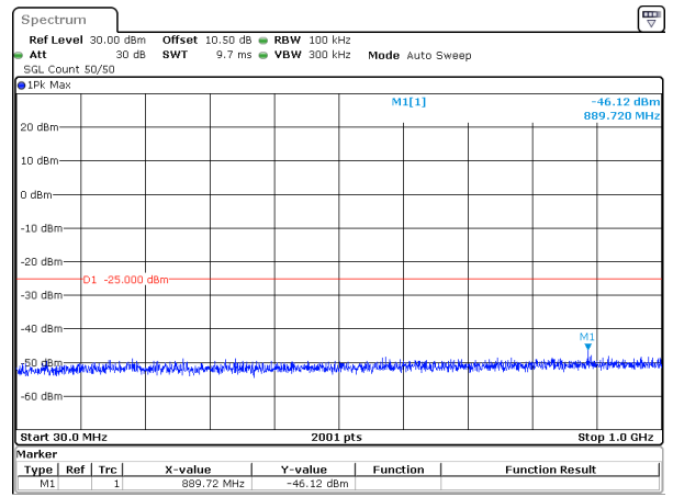
100MHz_30kHz_2640MHz_DFT-s-OFDM QPSK_RB1@0&-46.12 dBm
