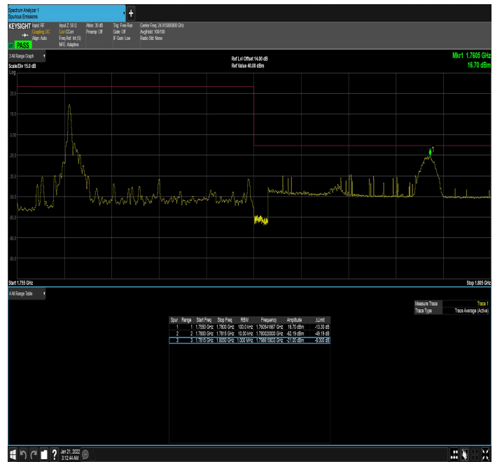
n66_20MHz_15kHz_1770MHz_DFT-s-OFDM QPSK_RB1@0
