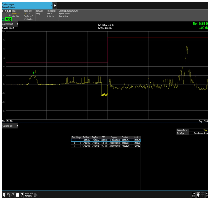
n66_20MHz_15kHz_1720MHz_DFT-s-OFDM QPSK_RB1@105
