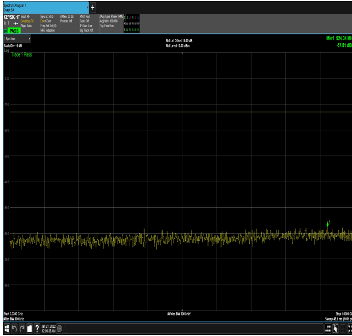
n66_10MHz_15kHz_1745MHz_DFT-s-OFDM QPSK_RB50@0|30MHz_1GHz
