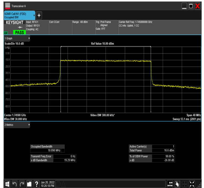
DC_12A_n66A_10MHz|20MHz_15kHz_707.5MHz|1745 MHz_QPSK|CP-OFDM 256 QAM_RB50@0|RB106@0
