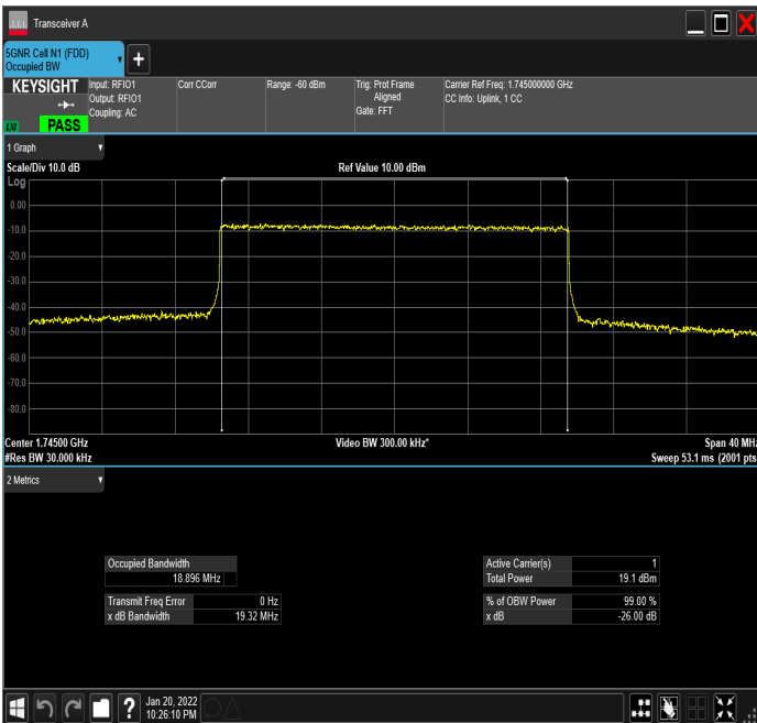
DC_12A_n66A_10MHz|20MHz_15kHz_707.5MHz|1745 MHz_QPSK|CP-OFDM 64 QAM_RB50@0|RB106@0
