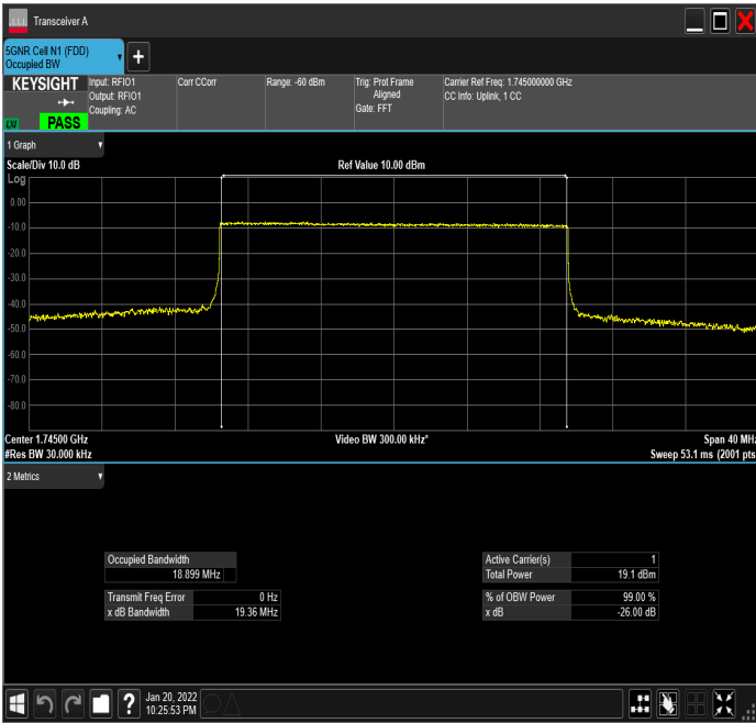
DC_12A_n66A_10MHz|20MHz_15kHz_707.5MHz|1745 MHz_QPSK|CP-OFDM QPSK_RB50@0|RB106@0
