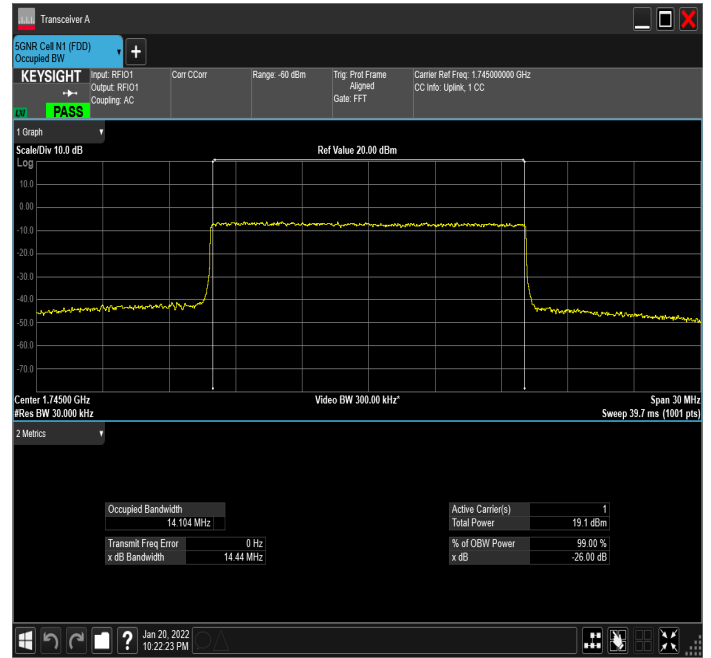
DC_12A_n66A_10MHz|15MHz_15kHz_707.5MHz|1745 MHz_QPSK|CP-OFDM 64 QAM_RB50@0|RB79@0
