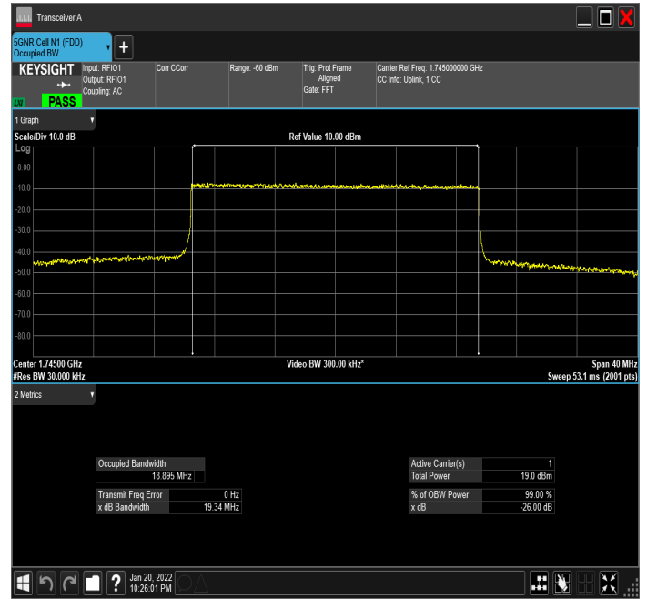
DC_12A_n66A_10MHz|20MHz_15kHz_707.5MHz|1745 MHz_QPSK|CP-OFDM 16 QAM_RB50@0|RB106@0
