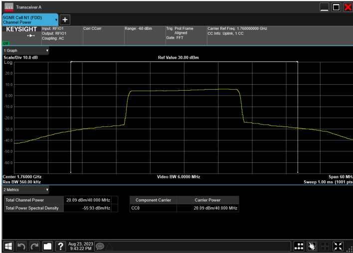
n66_40MHz_15kHz_1760MHz_CP-OFDM QPSK_RB216@0
