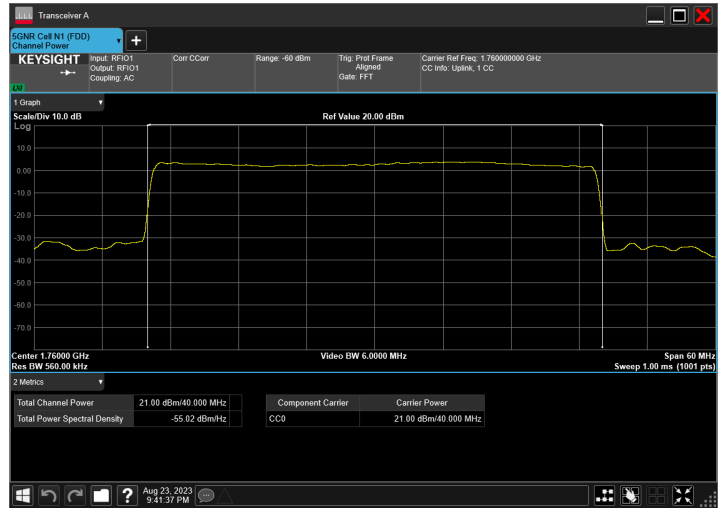
n66_40MHz_15kHz_1760MHz_DFT-s-OFDM PI/2 BPSK_RB216@0
