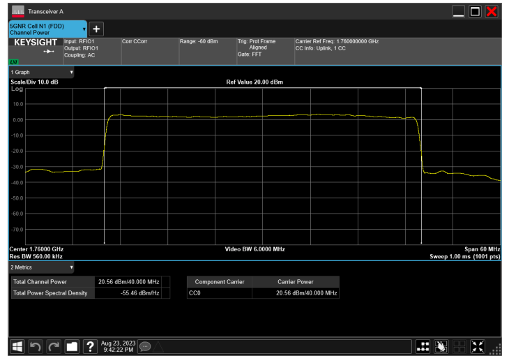
n66_40MHz_15kHz_1760MHz_DFT-s-OFDM QPSK_RB216@0
