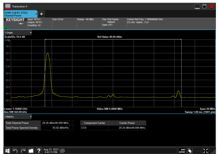
n66_40MHz_15kHz_1760MHz_CP-OFDM QPSK_RB1@1
