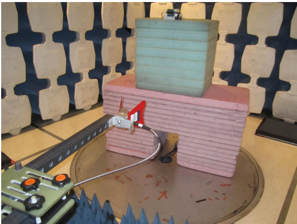
6-18GHz
