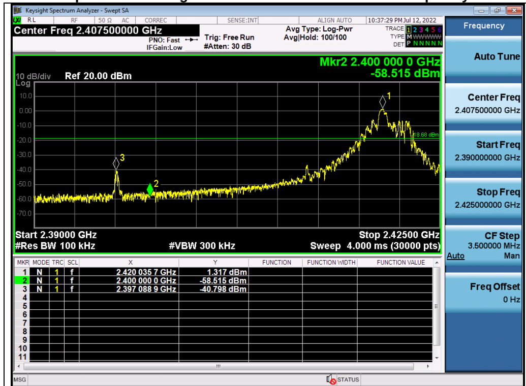
Test_Graph_GFSK_ANT1_2420_Lower Band Edge Emissions
