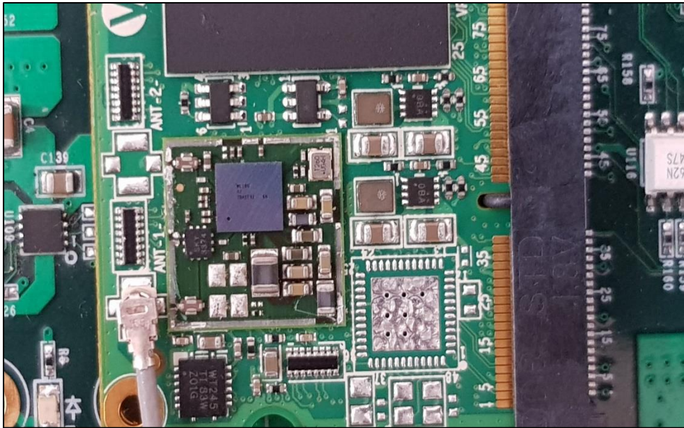
SOM PCBA_WiFi BT Module_Internal Picture
