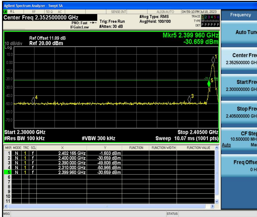
BLE_2M-Ant1-2402
