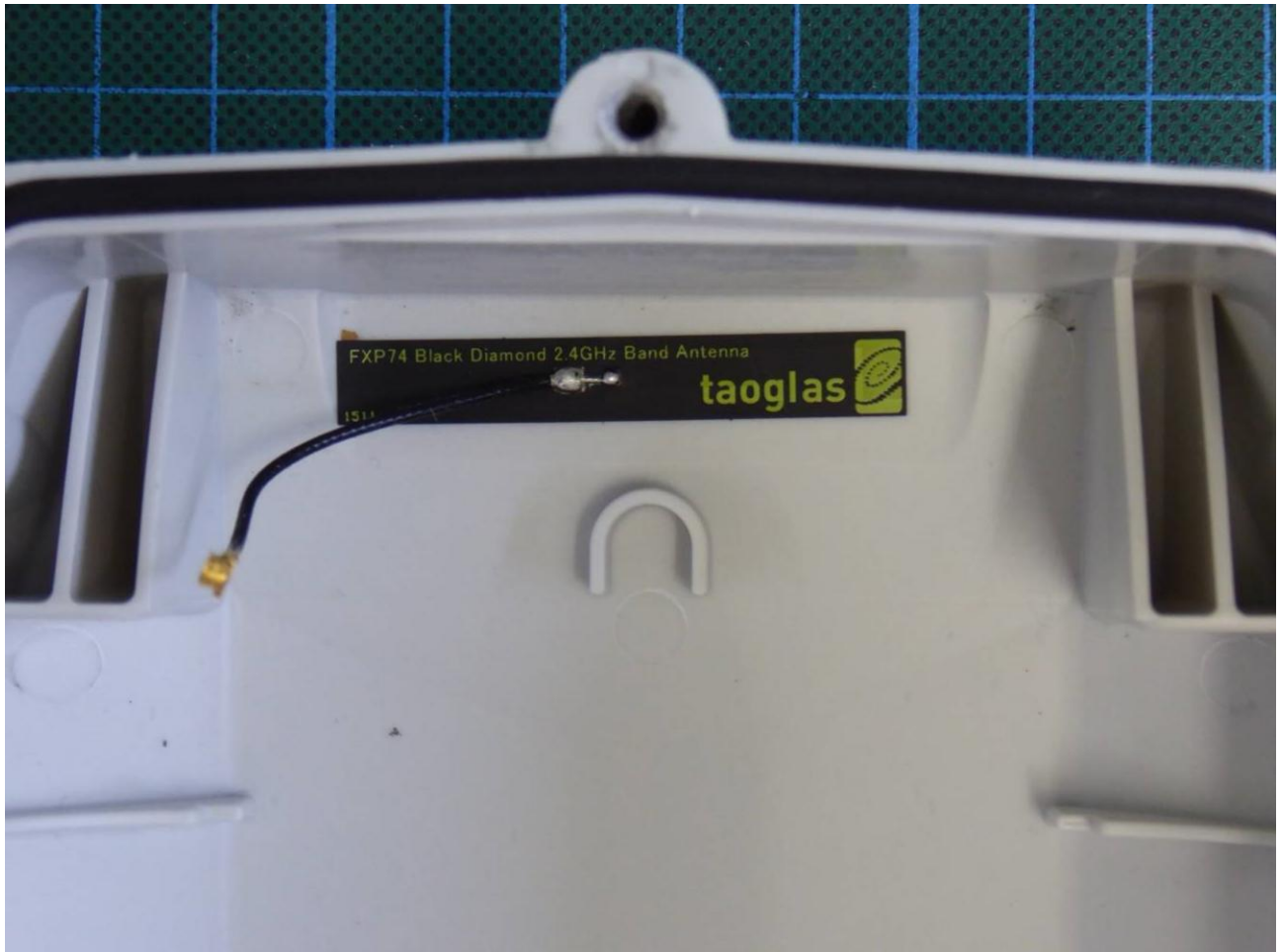
EUT 2.4 GHz antenna
