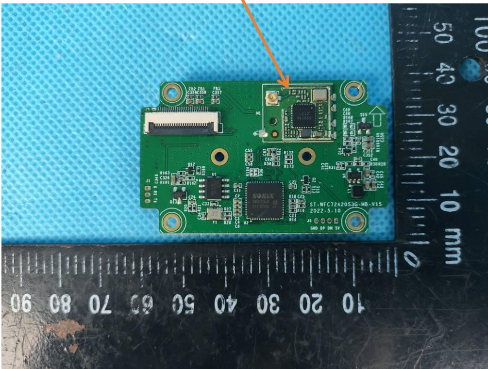
Wi-Fi Module
